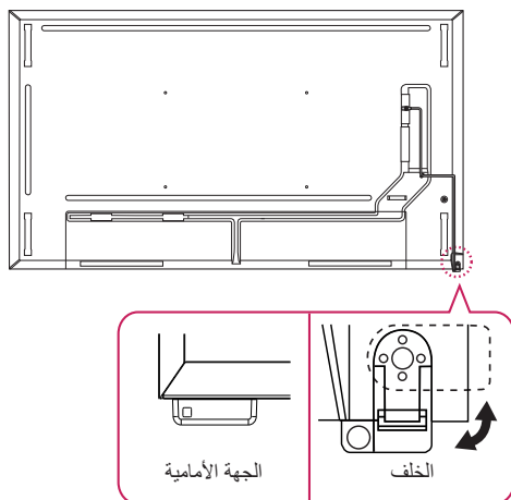
الاستخدام الأفقي (التركيب الافتراضي)
