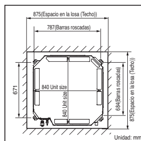
Chasis TM/TN/TP
