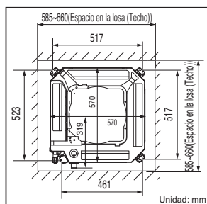
Chasis TQ/TR
