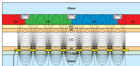
Échelle de pixels ITO ou MoTi
