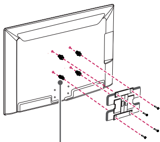
Espaceurs internes pour fixation murale
