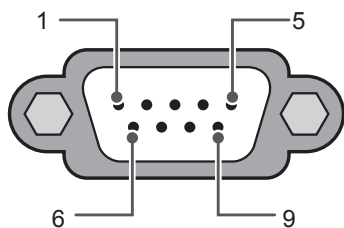
RS-232C (Puerto serie)
