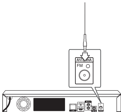
Заден панел на устройството
