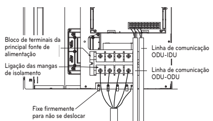
Conexão de comunicação
