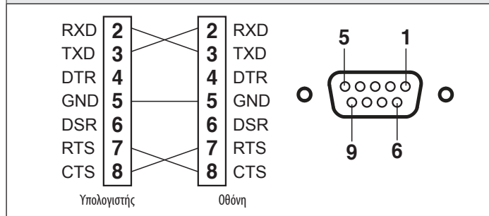
Εικόνα 1: Διάγραμμα σύνδεσης RS-232C
