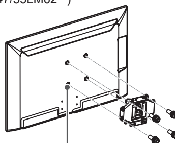
Entretoise intérieure pour montage mural (selon le modèle)
