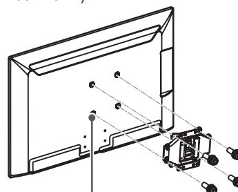
Inneres Distanzstück für Wandhalterung (Abhängig vom Modell)
