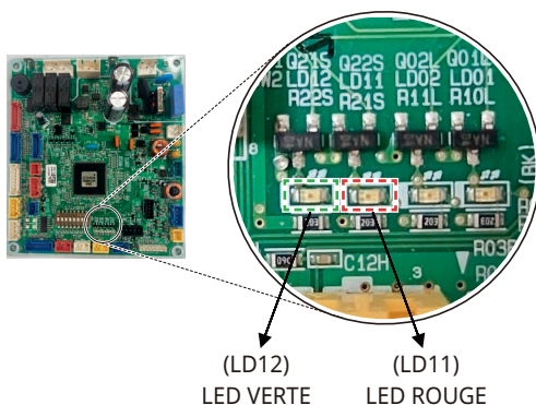
2. Type de circuit imprimé principal (Le sous-PCB du capteur R32 est intégré dans le circuit imprimé principal)
