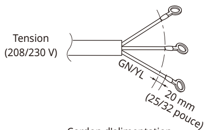
Cordon d'alimentation
