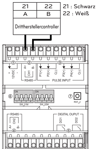
Zählerschnittstelle
