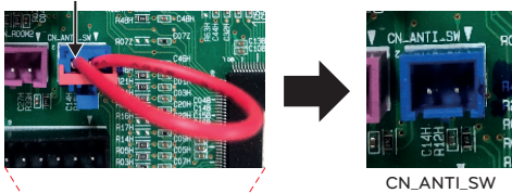
CN_ANTI_SW
