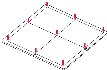
Общая нагрузка: 300 кг на окне детектора
