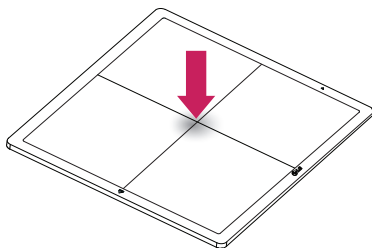
Частичная нагрузка: 100 кг в центральной части диаметром 40 мм
