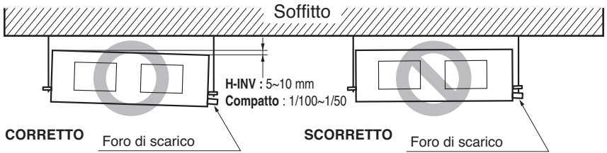
Condotto nascosto nel soffitto - H-INV (Inverter alto), Compatto
