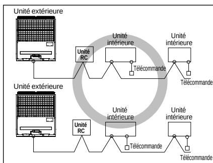
Câble 2-brins isolé
