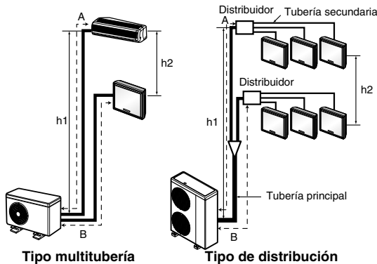
Tipo multitubería
