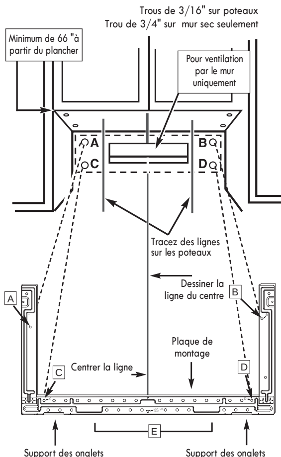
Plaque de montage de 3 pièces
