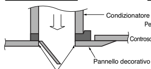
Corretta installazione
