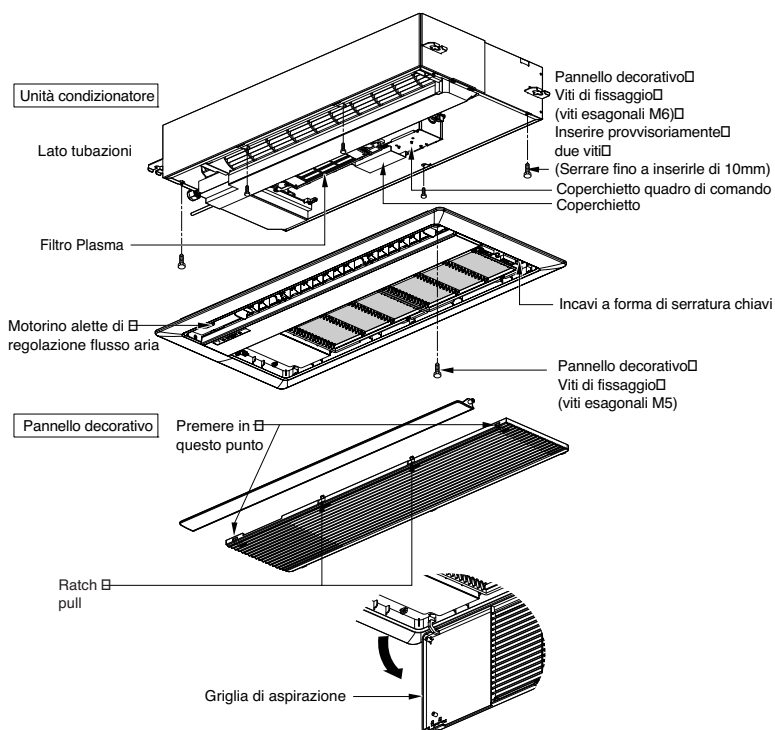
Corretta installazione
