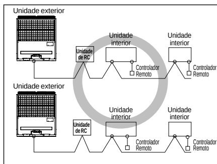
Cabo blindado de 2 condutores
