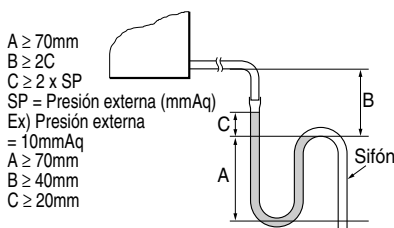
Dimensiones del sifón
