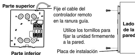
<Parte frontal de la placa de instalación>
