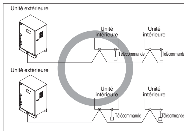
Câble bipolaire blindé
