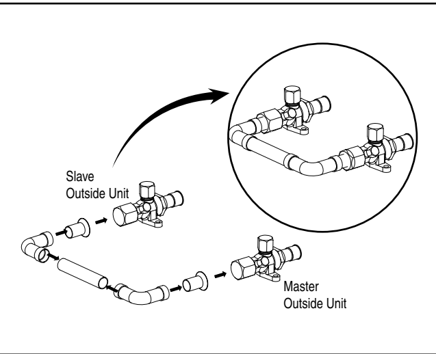
2 unités extérieures
