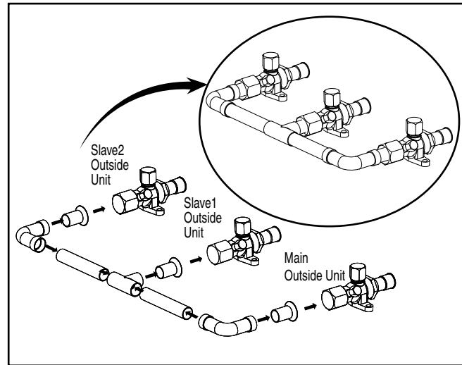
3 unités extérieures
