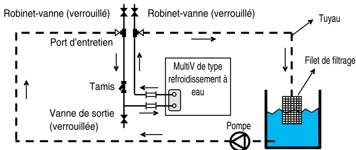
[Nettoyage de l'échangeur de chaleur radiant]
