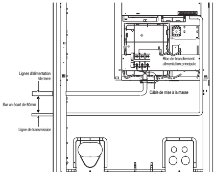
Côté gauche
