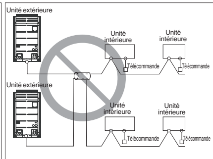
Câble multipolaire
