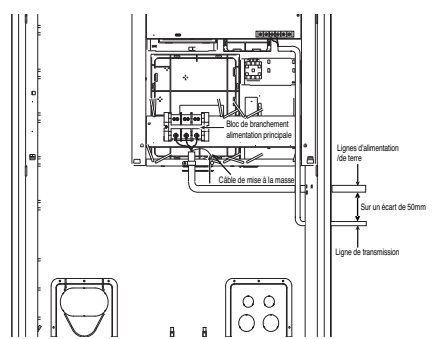
Côté droit
