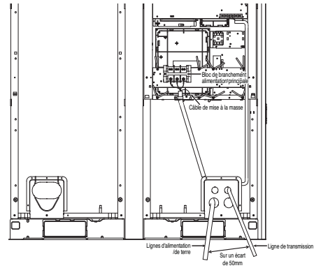
Façade avant 2
