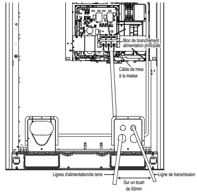
Façade avant 2
