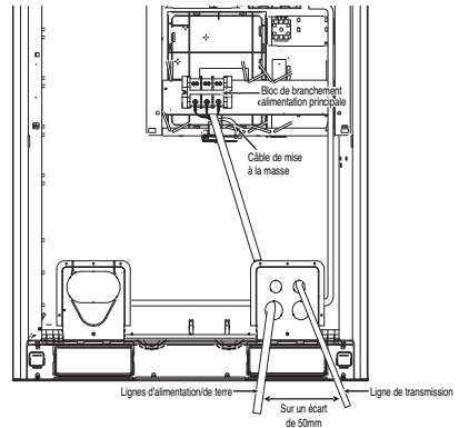
Façade avant 2
