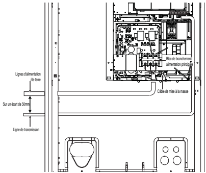
Côté gauche
