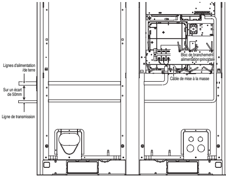
Façade avant 1
