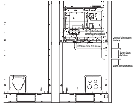
Façade avant 2
