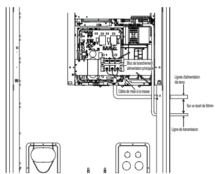
Côté droit
