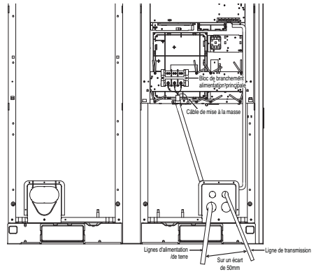
Façade avant 2
