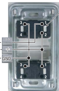
< Côté arrière de contact sec de l'unité extérieure >
