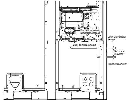
Façade avant 2
