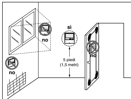
Fig. 1 Posizioni tipiche per il telecomando
