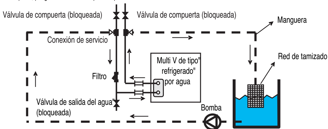
[Limpieza del intercambiador de calor de paneles]
