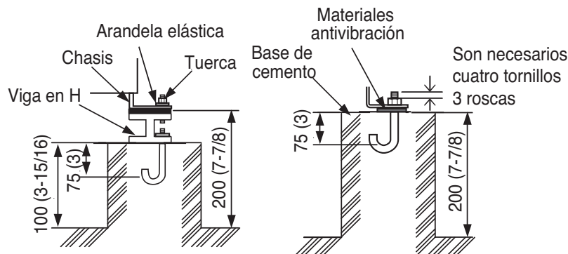
Método de atornillado de base
