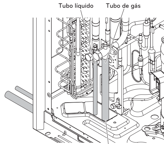
Retire apenas líquido / tubulação de gás Knock Out
