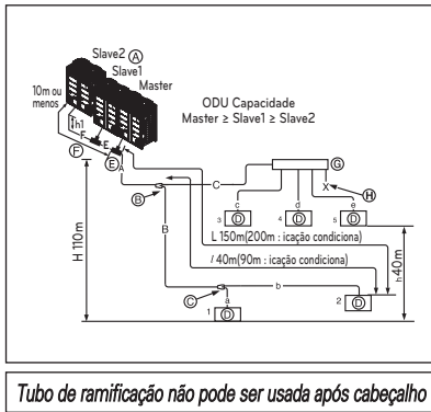
(Tabela 1) Comprimento limite do tubo
