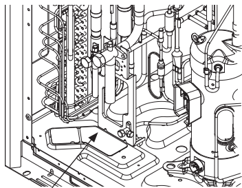
Área de Extracción de Líquido / tubos conexiones laterales inferiores de gas.
