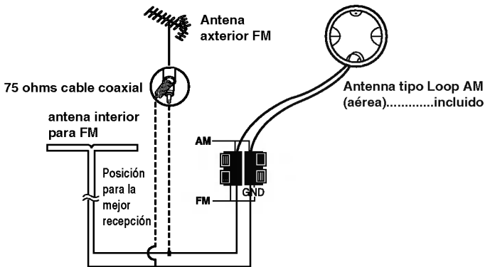
(1) 2 BANDA (FM/AM) aérea
