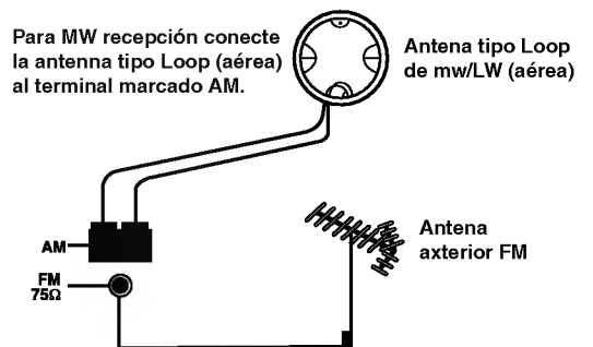
(4) 2 BANDA [(FM/AM(MW))] aérea
