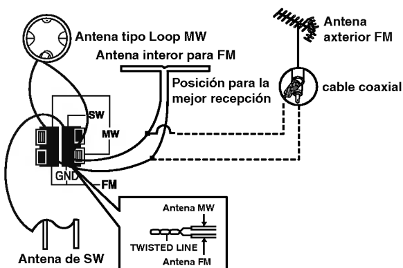
(3) 3 BANDA (FM/MW/SW) aérea
