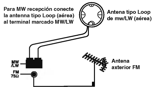
(4) 2 BANDA [(FM/AM(MW))] aérea
