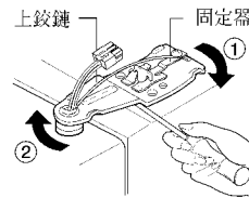
上鉸鏈
