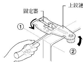
上鉸鏈
