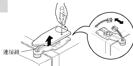
上鉸鏈
