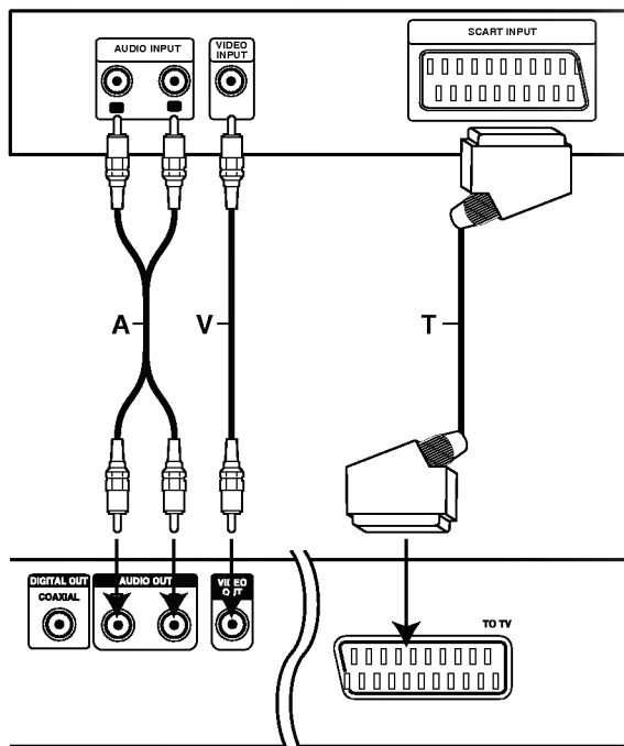
Parte trasera del reproductor de DVD
