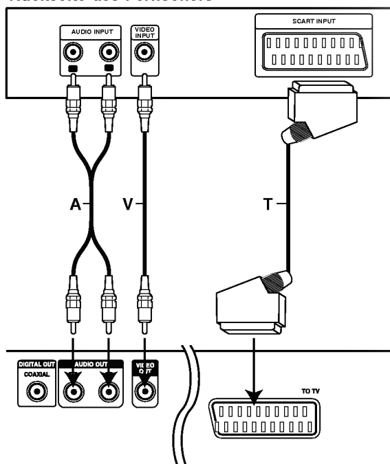
Rückseite des DVD-Spielers
