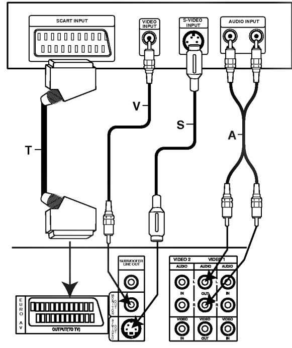
Parte posterior del receptor de DVD/CD
