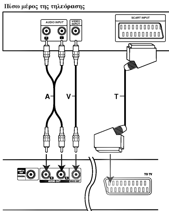
Πίσω μέρος της τηλεόρασης Πίσω μέρος του DVD Player
