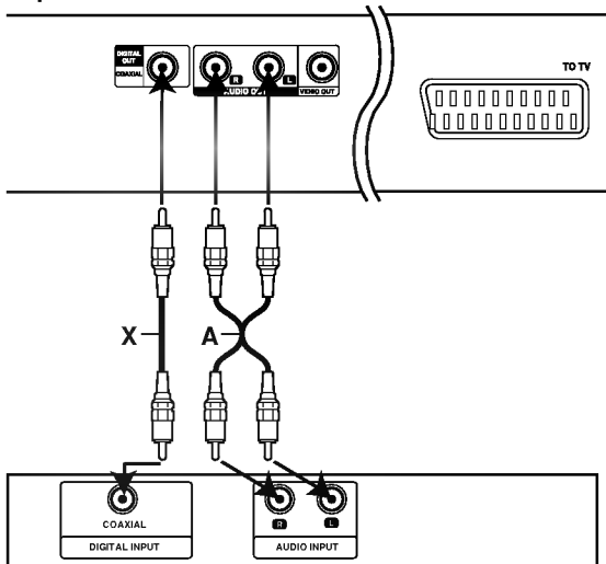
Amplificador (Receptor)
