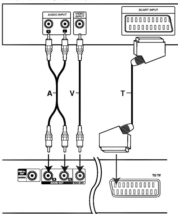
Partie arrière du Lecteur DVD
