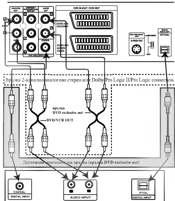
Усилвател (Приемник)
