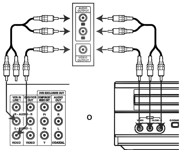
Parte trasera del DVD+VCR
