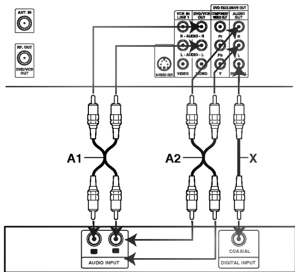
Amplificador (Receptor)
