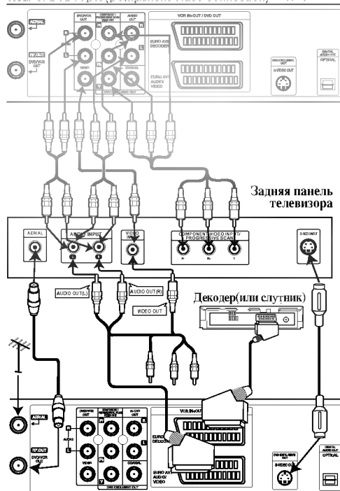
Задняя стенка прибора (простое соединение)
