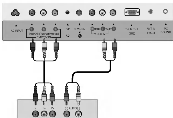
Decodificador de señales DTV
