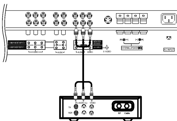
Cable Box
