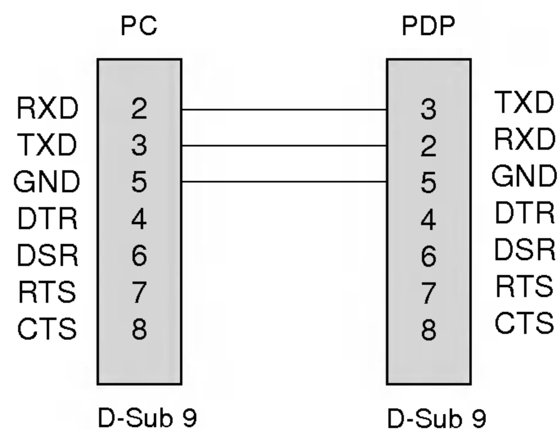
Configuración del cable de 3-alambres (No estándar)
