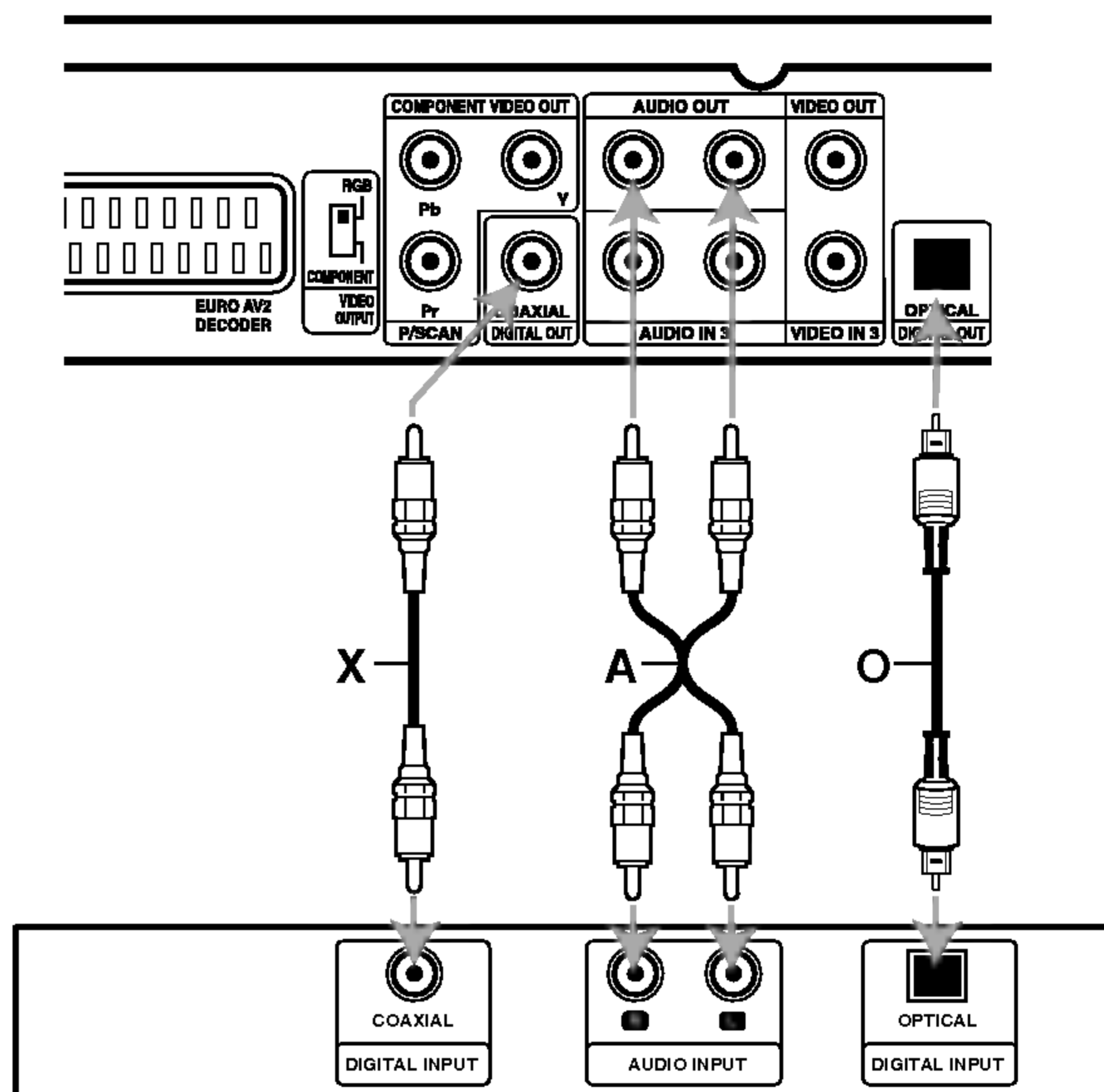
Усилвател (Приемник)
