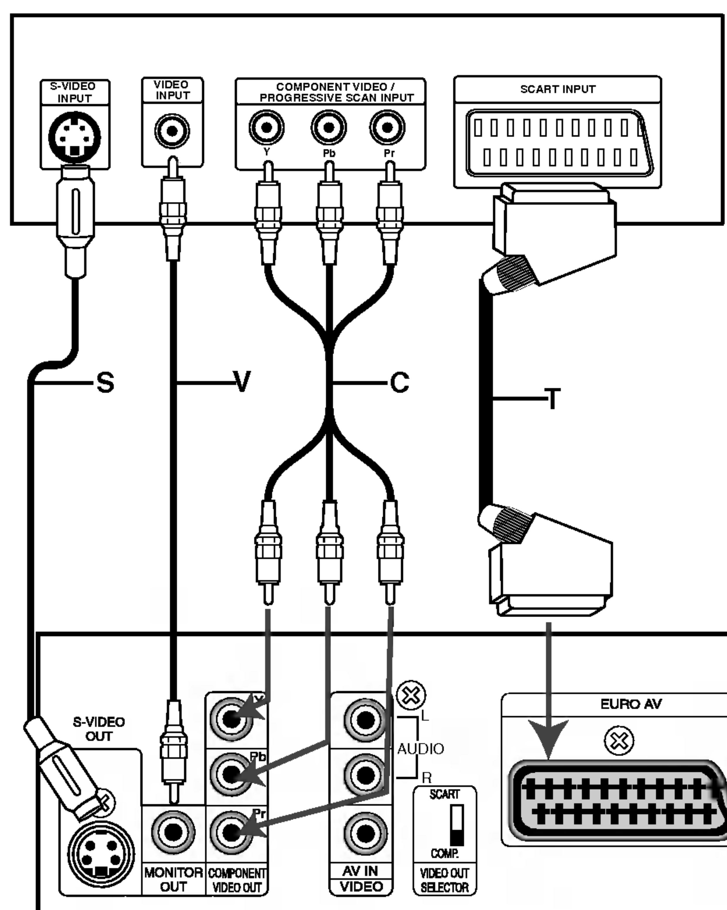
Panneau arrière du récepteur DVD/CD
