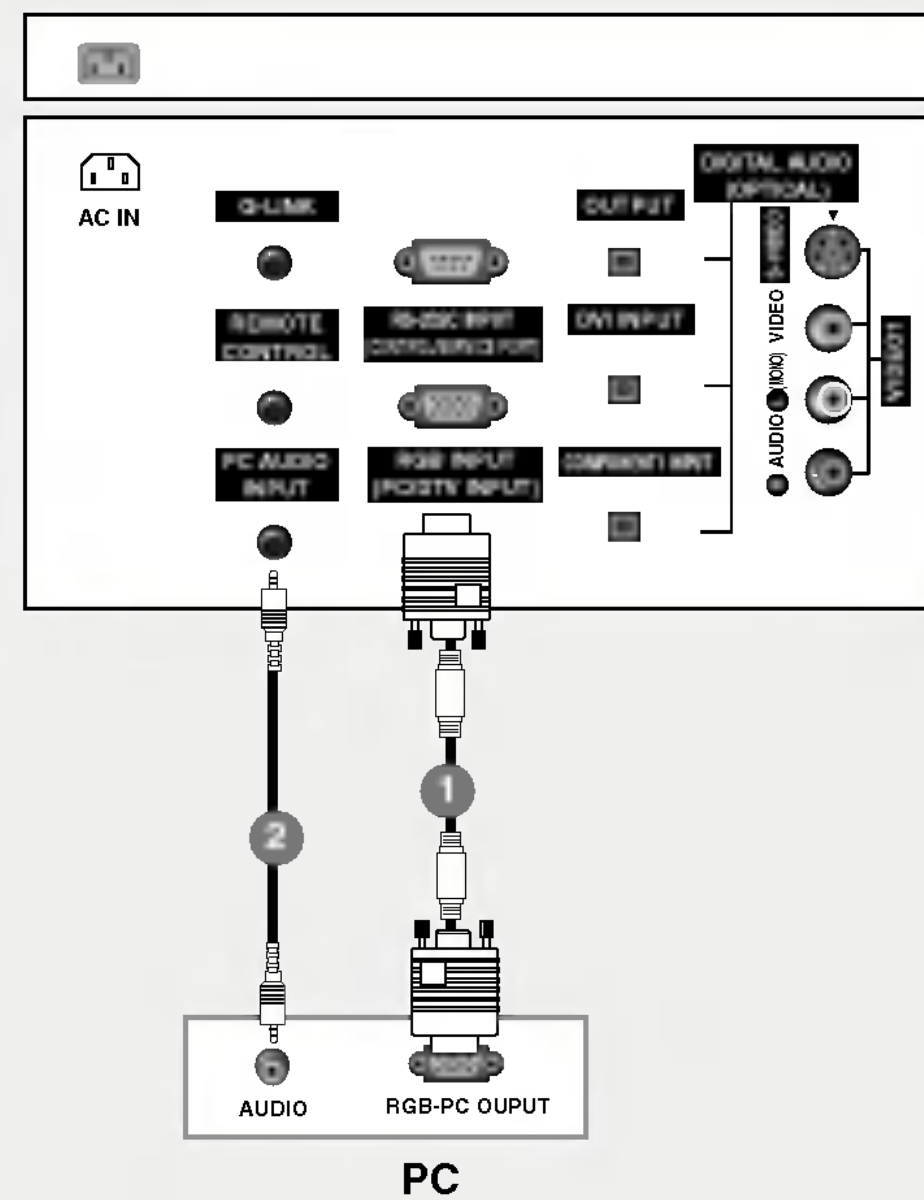
Arrière du téléviseur de 26 pouces
