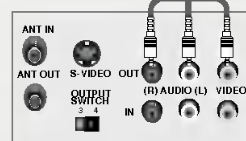
VCR (magnétoscope)
