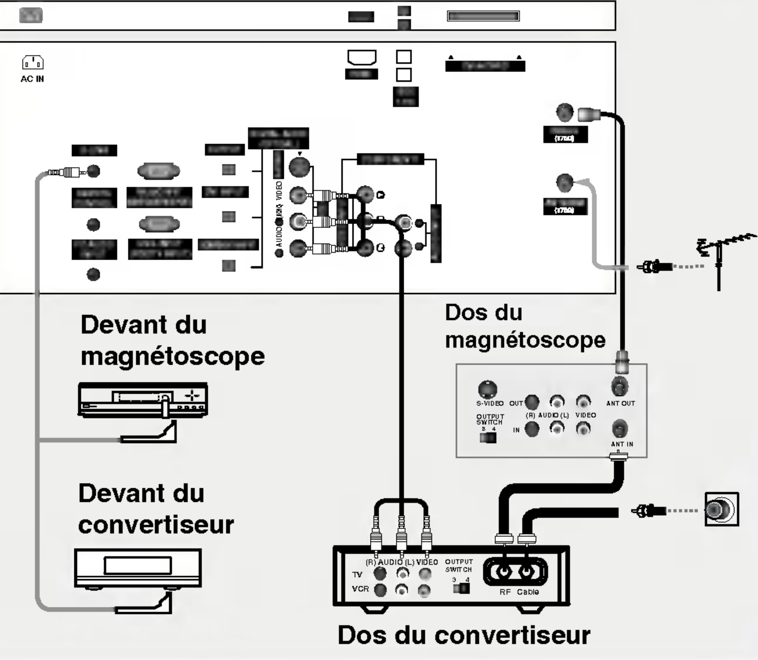
Arrière du téléviseur de 26 pouces
