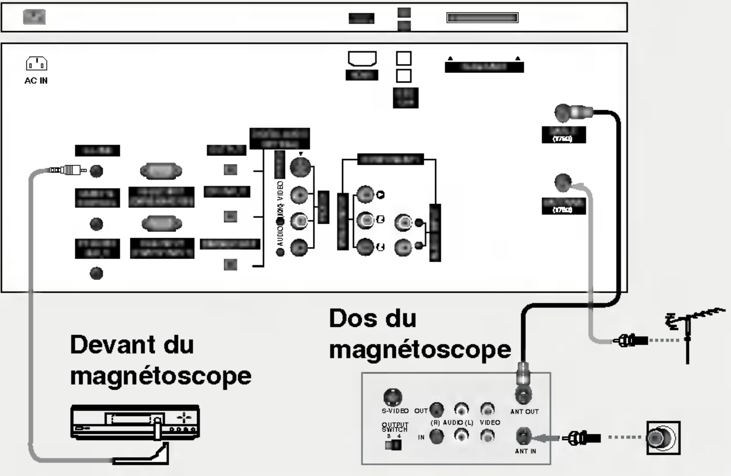
Arrière du téléviseur de 26 pouces
