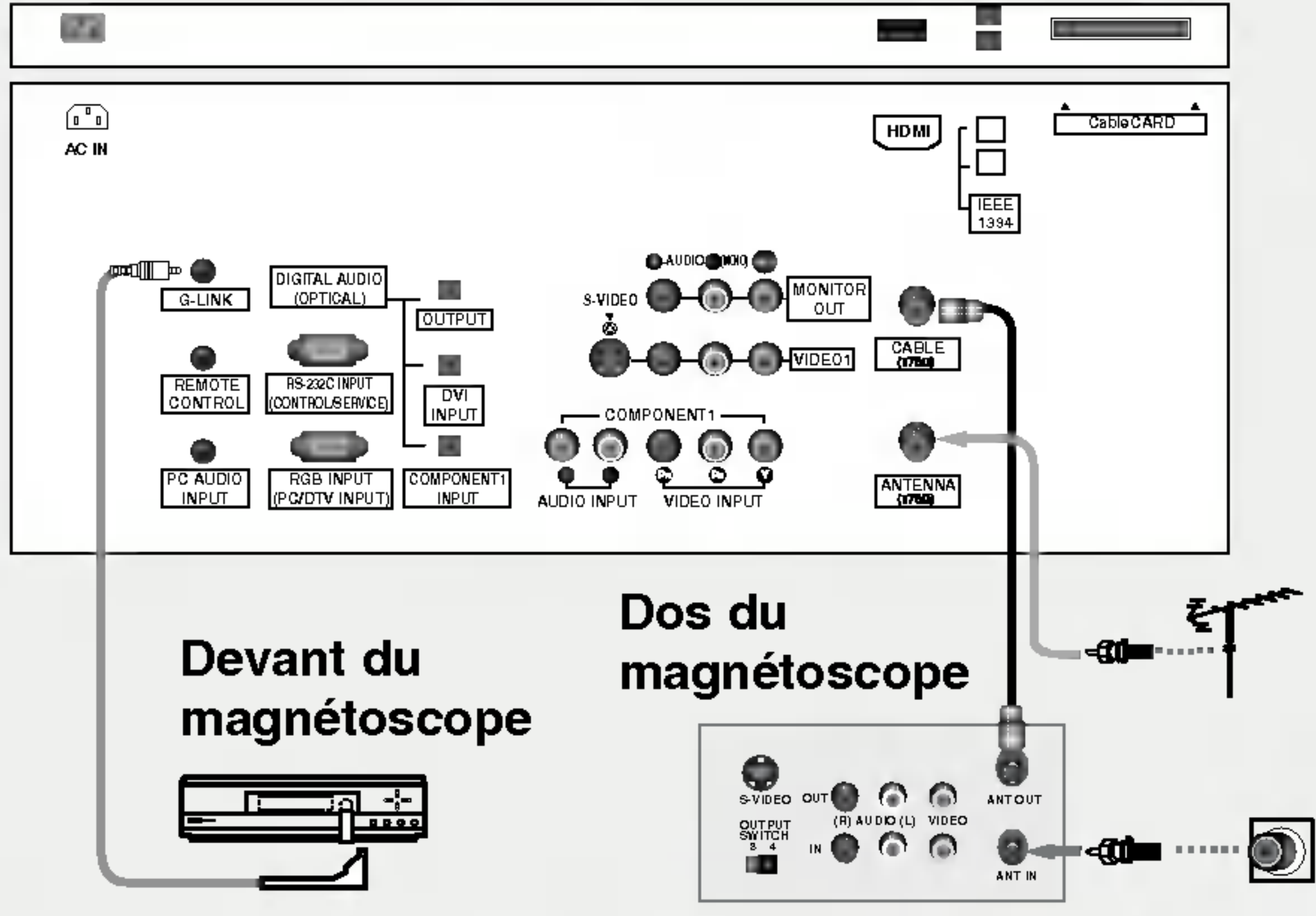
Arrière du téléviseur de 32, 37 et 42 pouces
