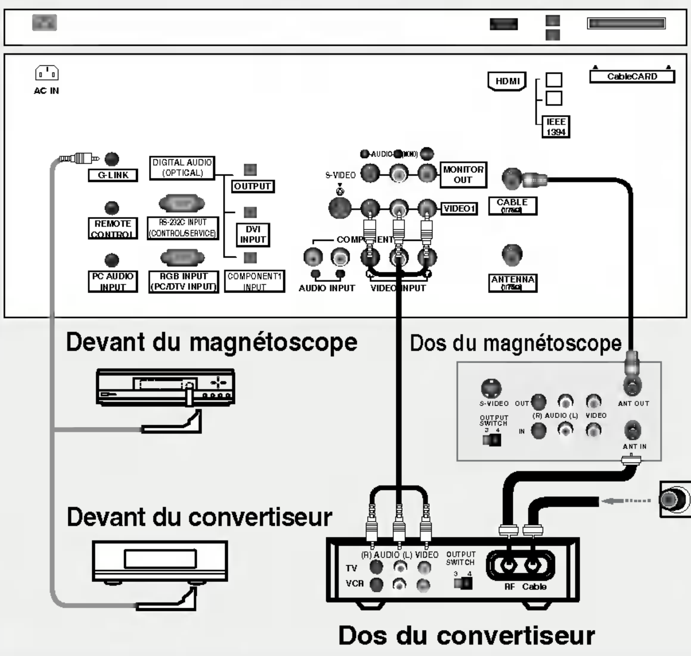
Arrière du téléviseur de 32, 37 et 42 pouces
