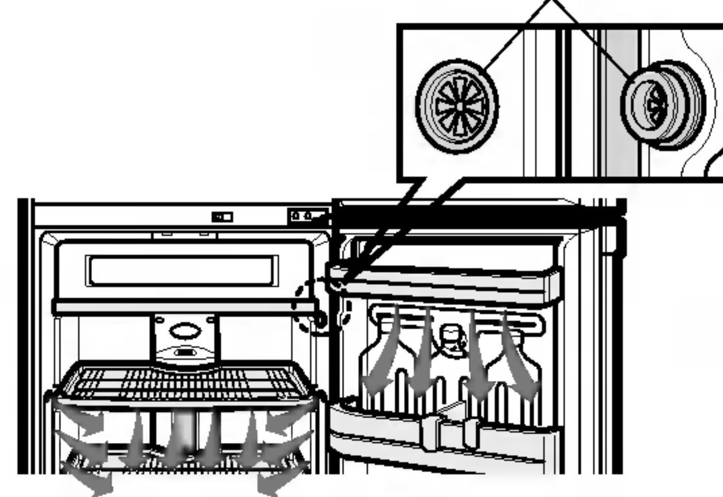
Camino de circulación de aire frío
