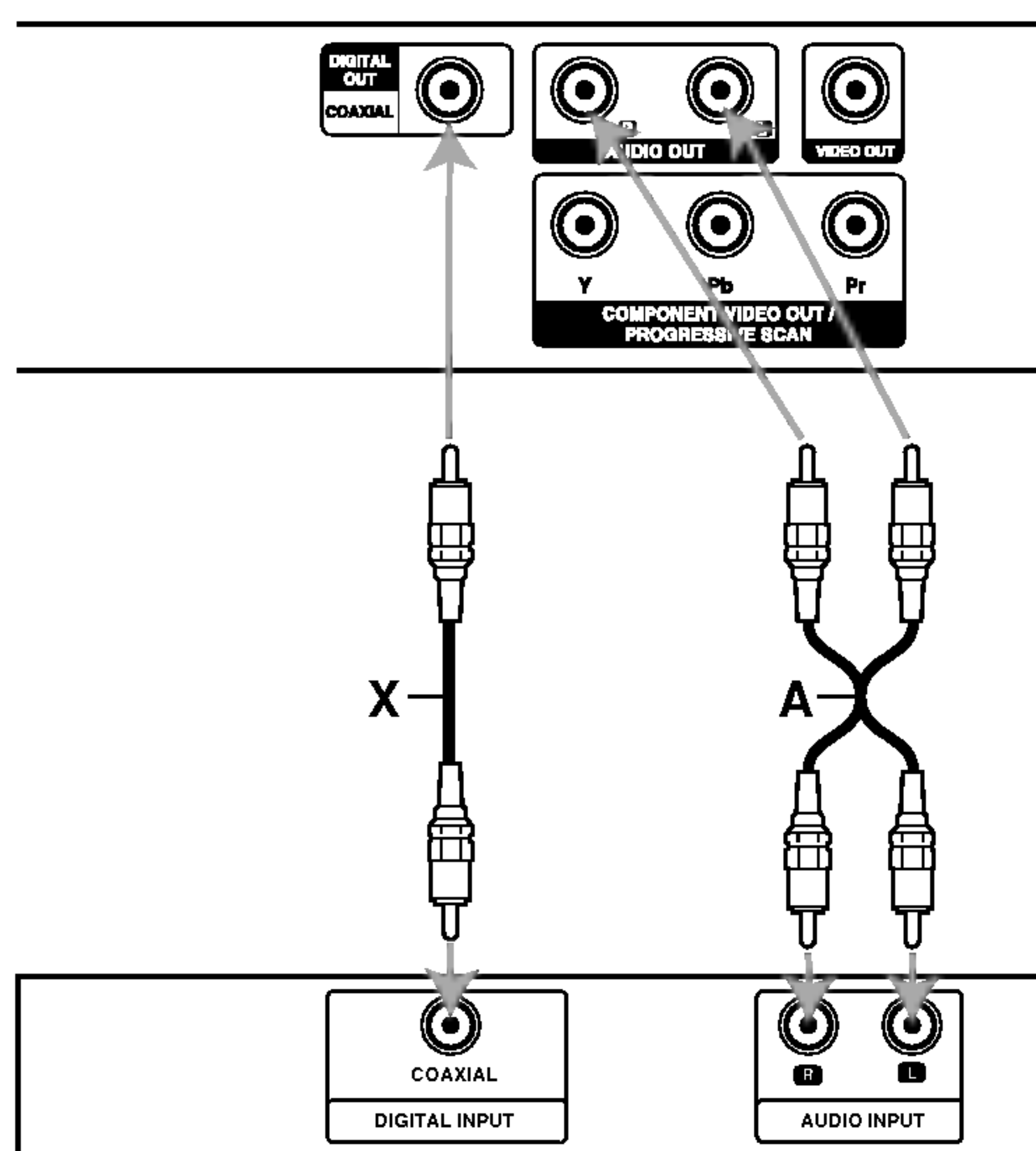
Erősítő (Rádióerősítő)
