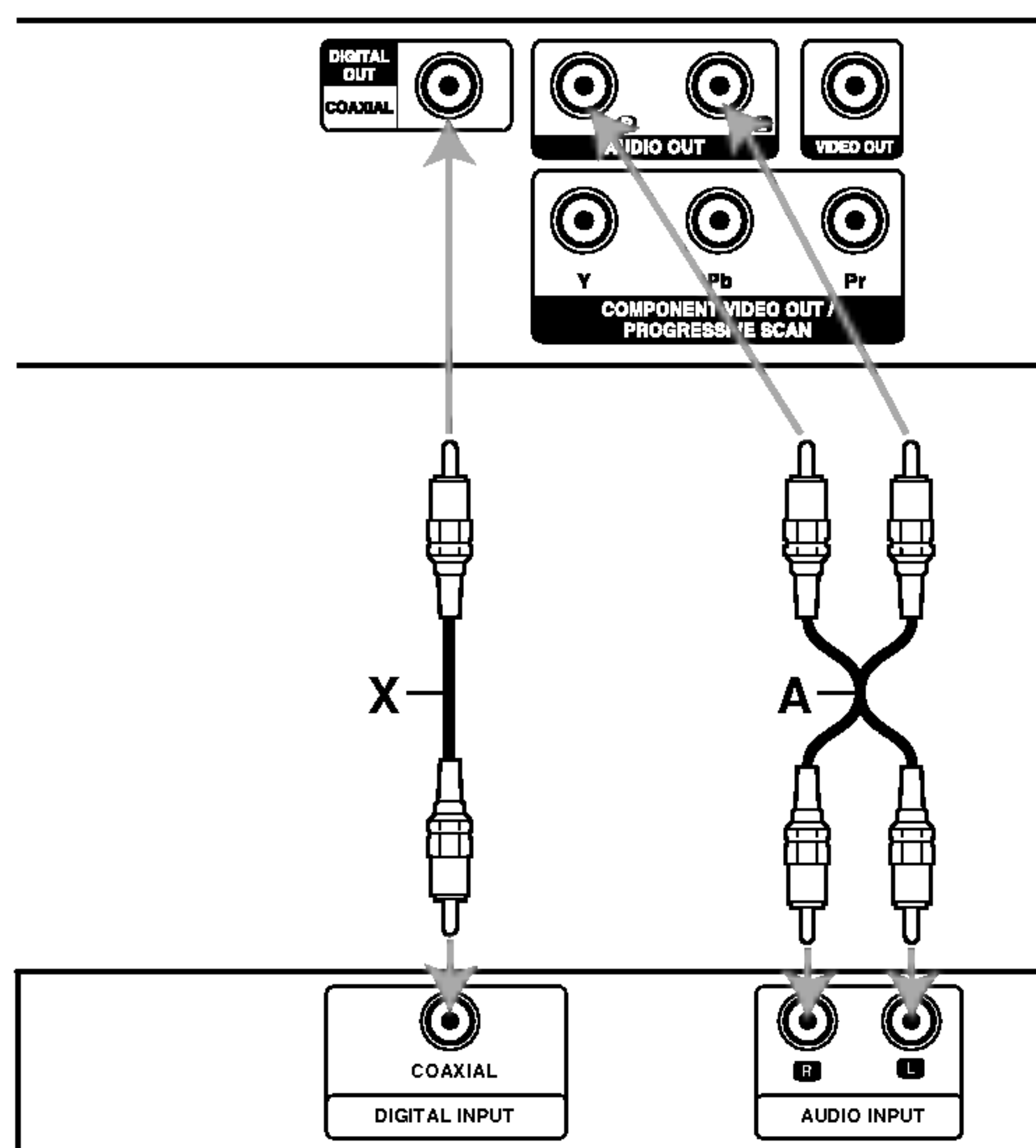
Зајакнувач (Рисивер)
