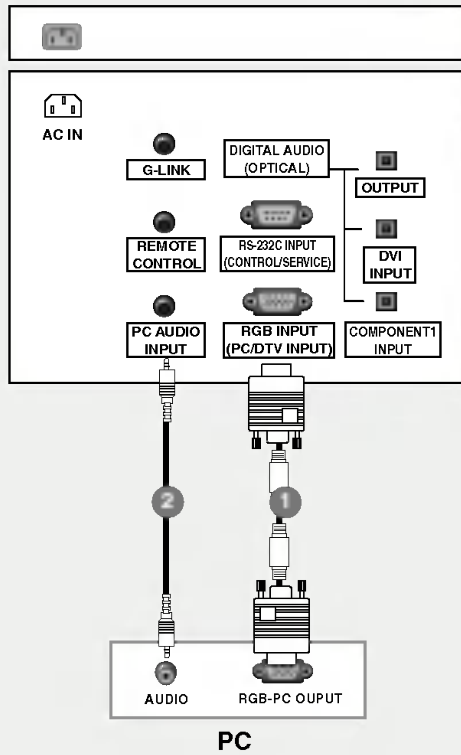
Arrière du téléviseur de 32, 37 et 42 pouces
