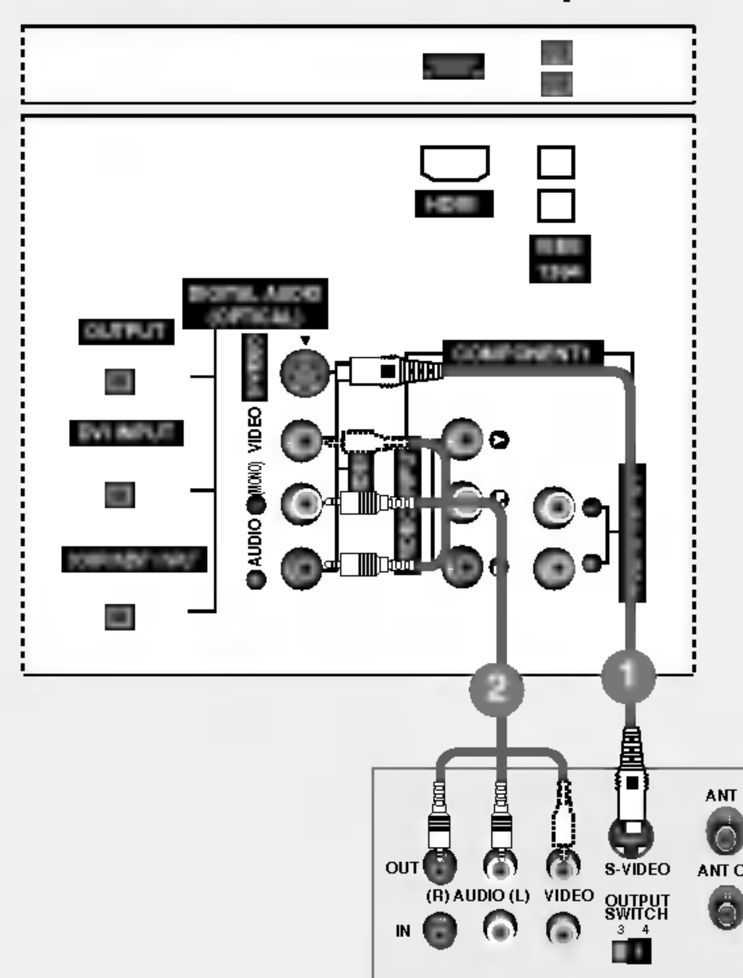
Arrière du téléviseur de 26 pouces
