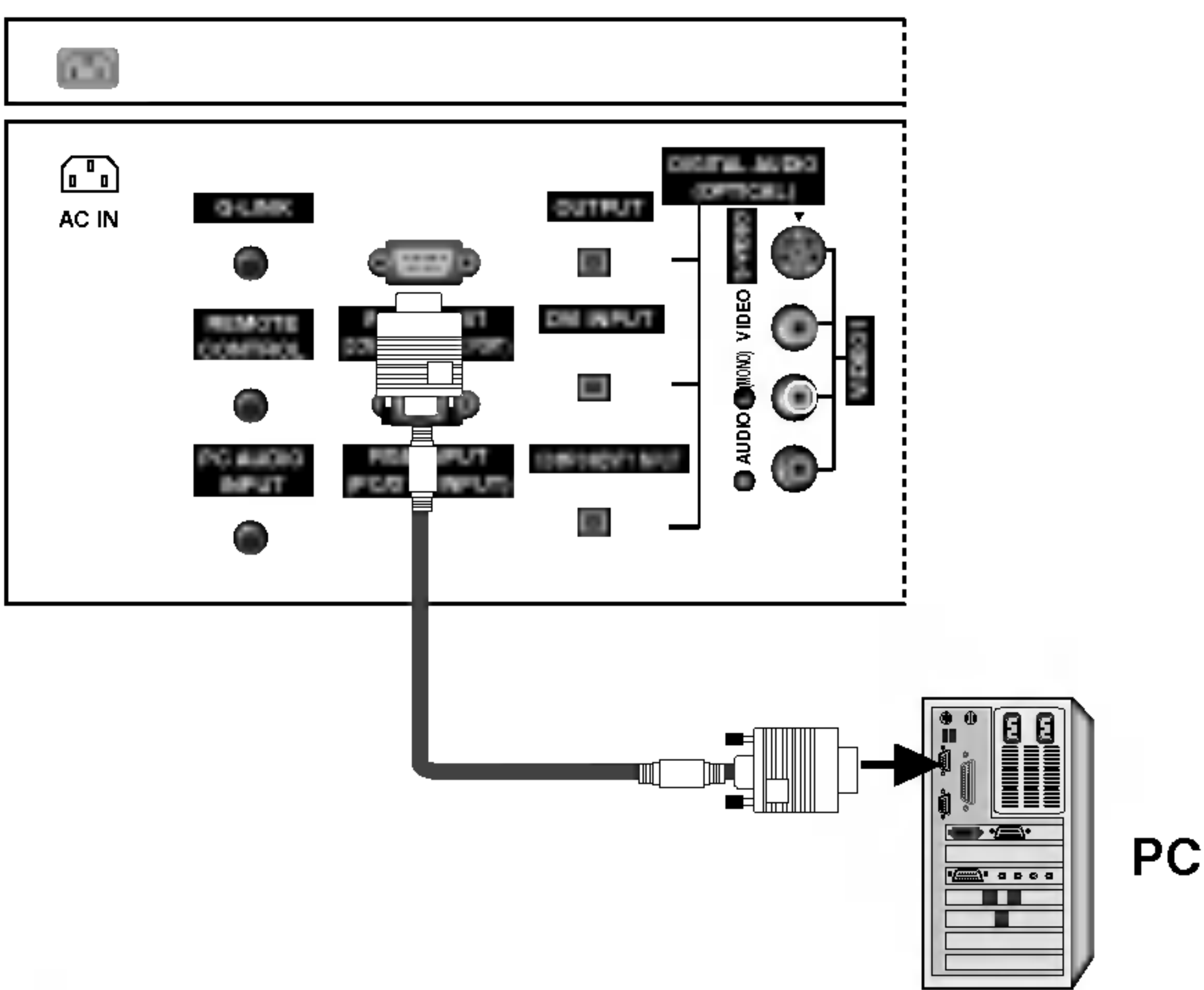
Arrière du téléviseur de 26 pouces
