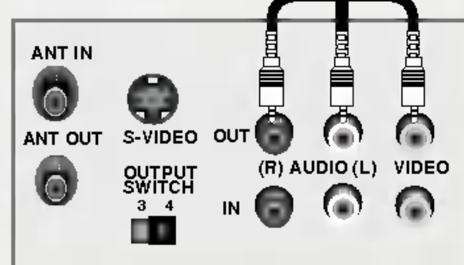
VCR (magnétoscope)
