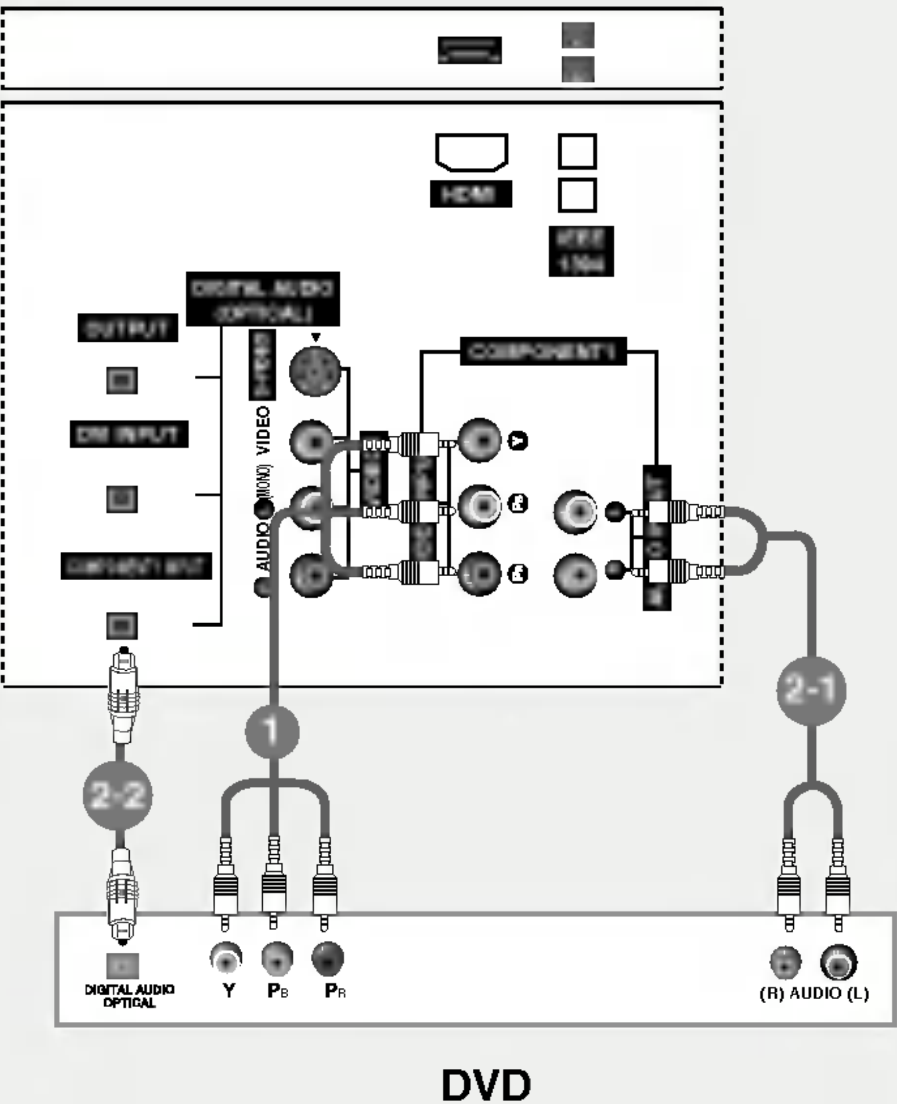
Arrière du téléviseur de 26 pouces
