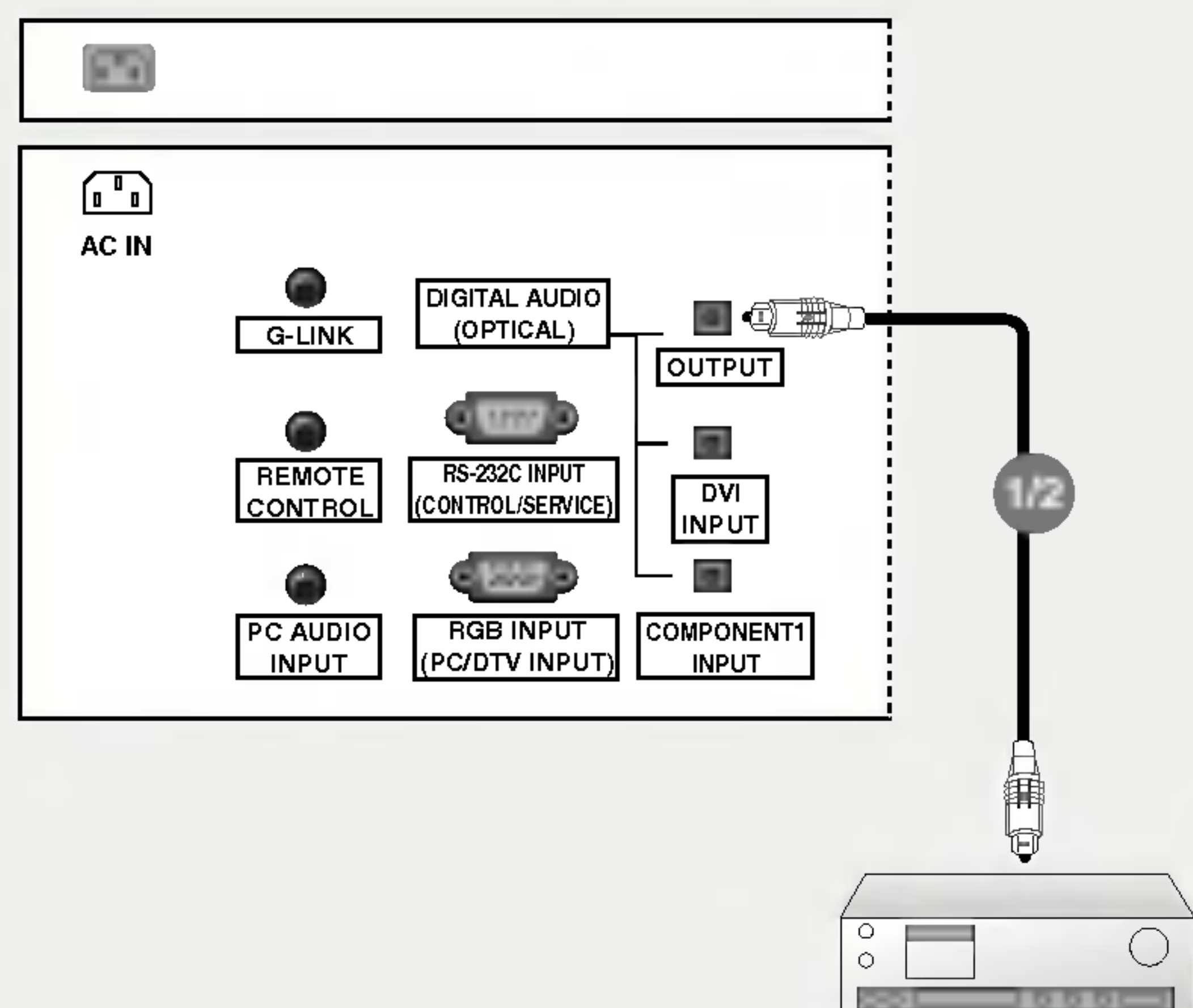
Arrière du téléviseur de 32, 37 et 42 pouces
