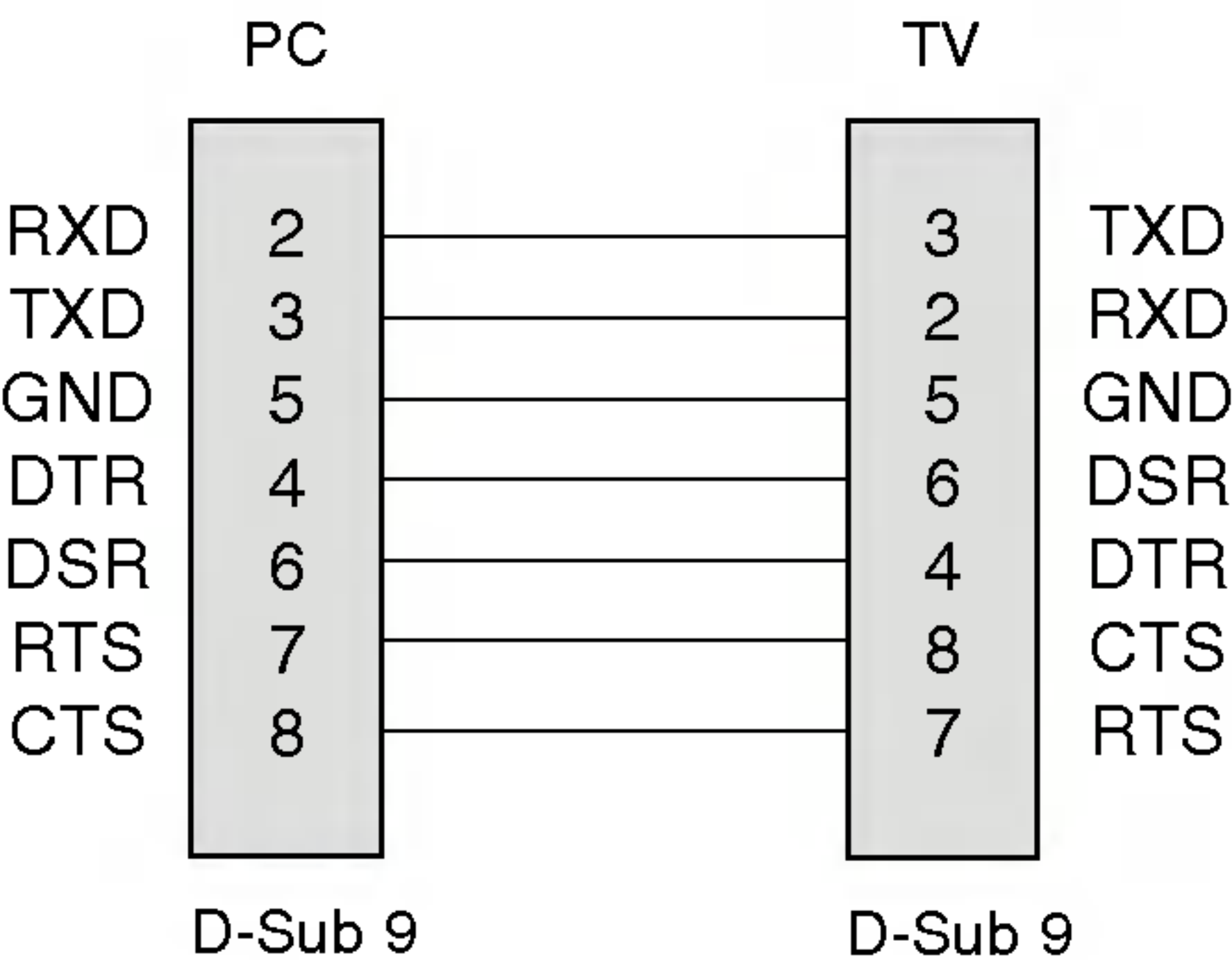
7-Configurations du câble (Câble simulateur de modem (série) avec connecteurs femelle-femelle)
