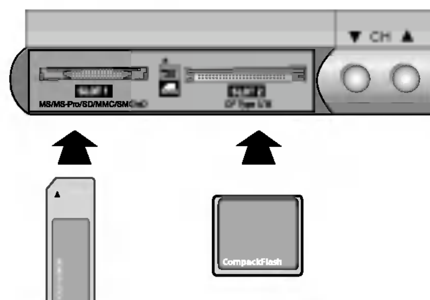
Panneau avant des modèles 32/37/42LP1D
