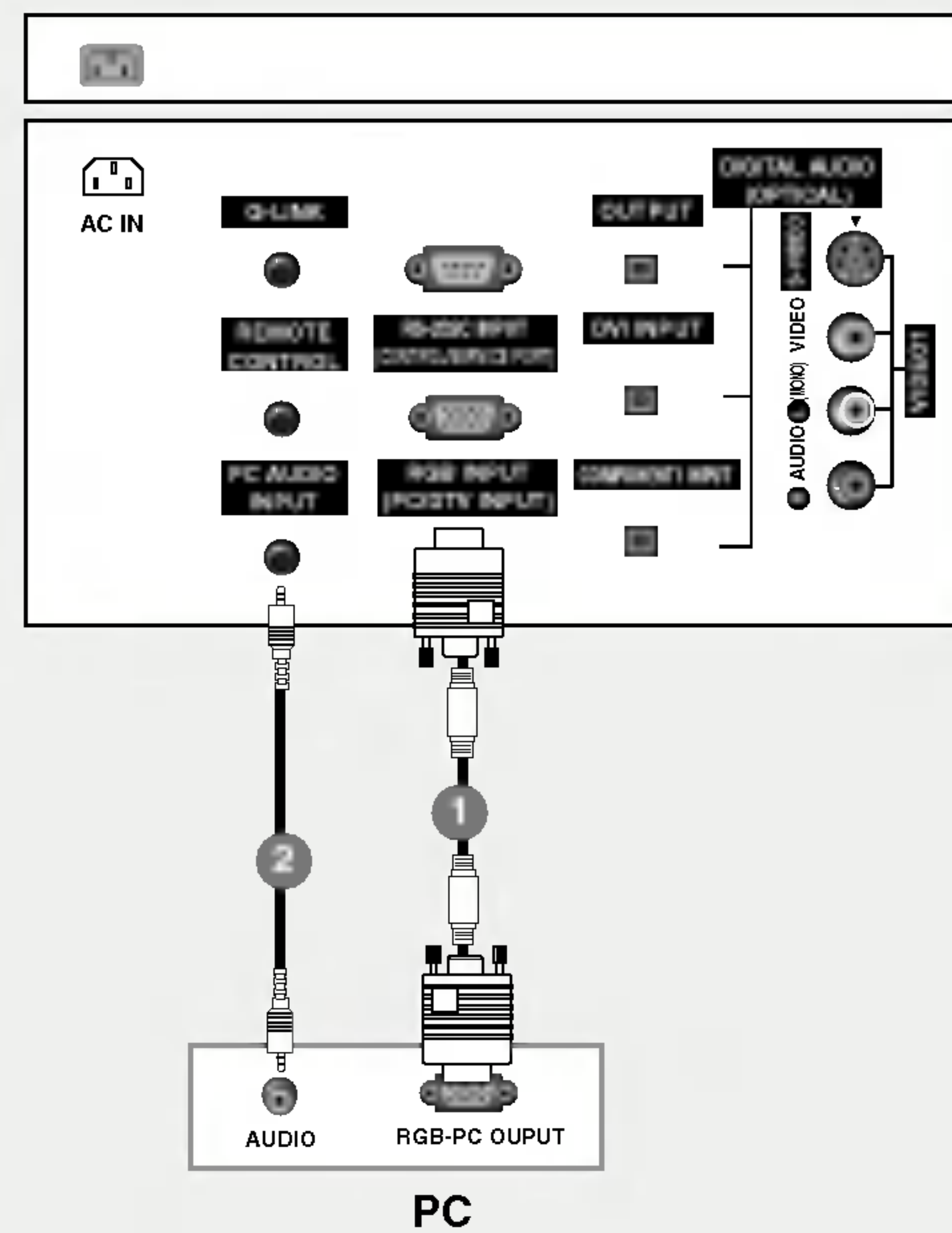
Arrière du téléviseur de 26 pouces
