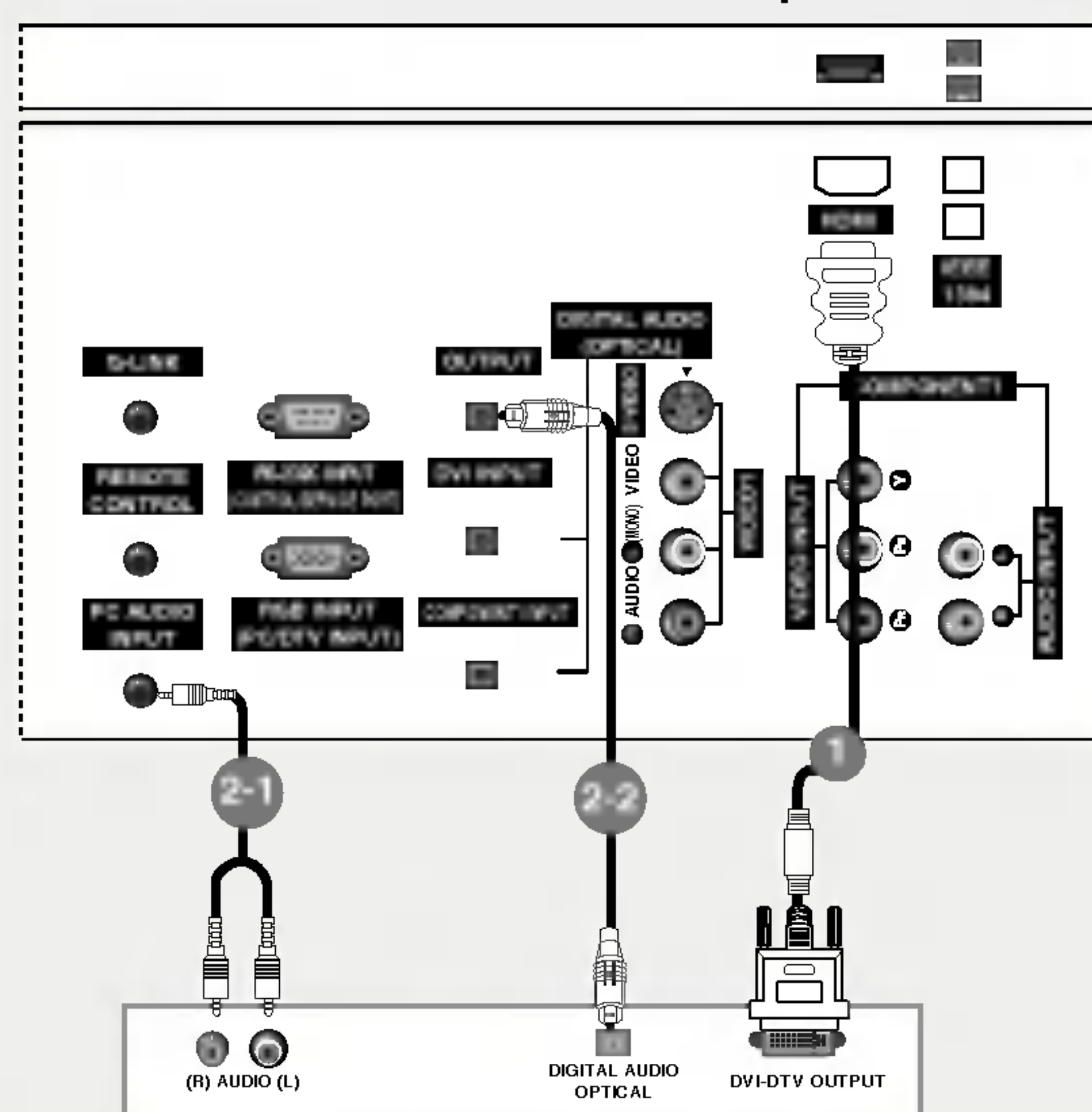
Boîtier décodeur numérique
