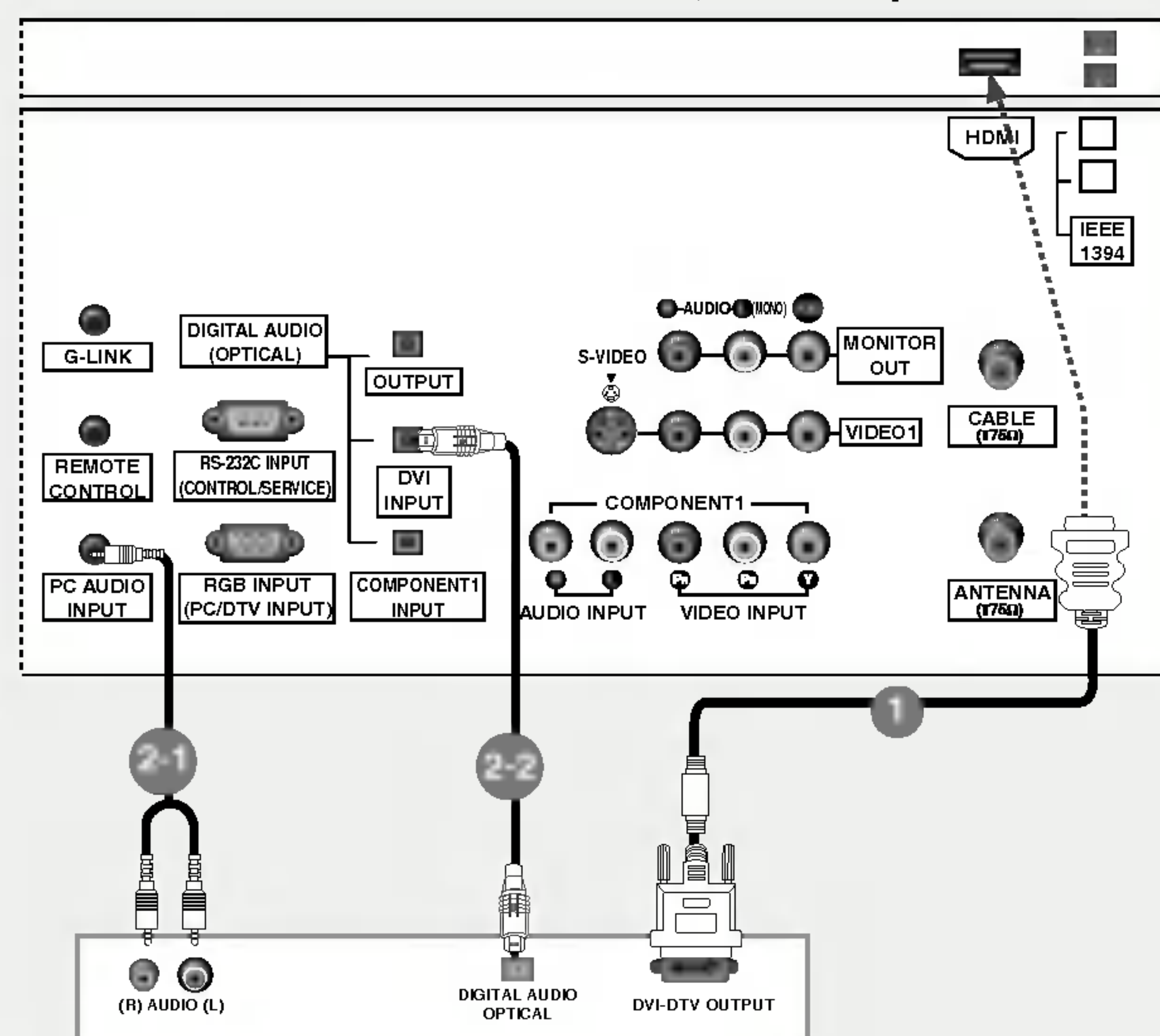
Boîtier décodeur numérique
