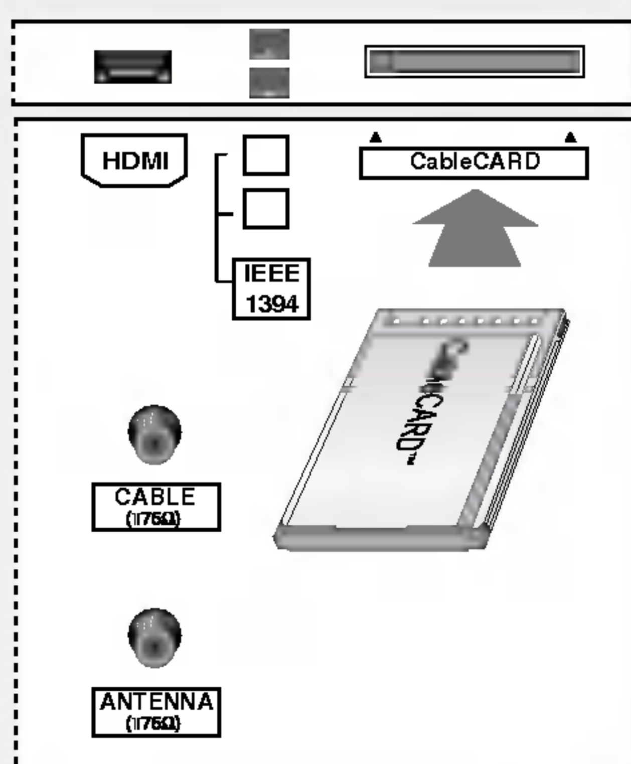
Arrière du téléviseur de 32, 37 et 42 pouces
