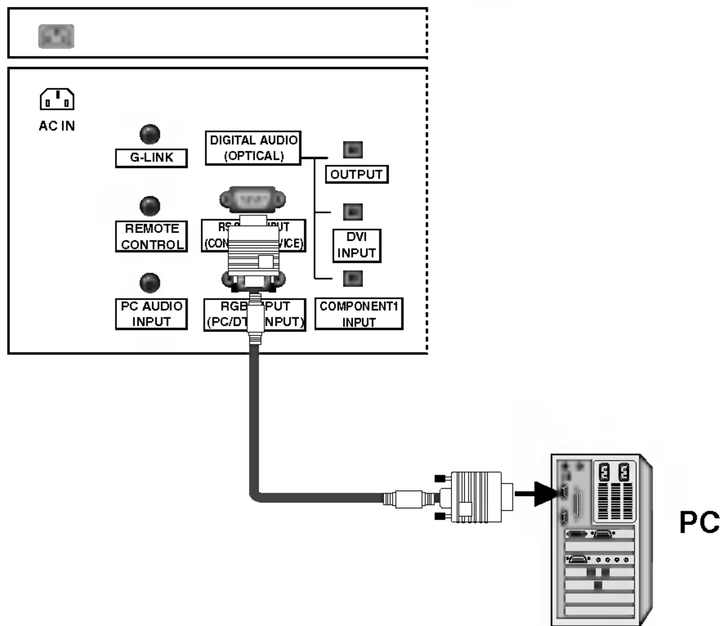
Arrière du téléviseur de 32, 37 et 42 pouces
