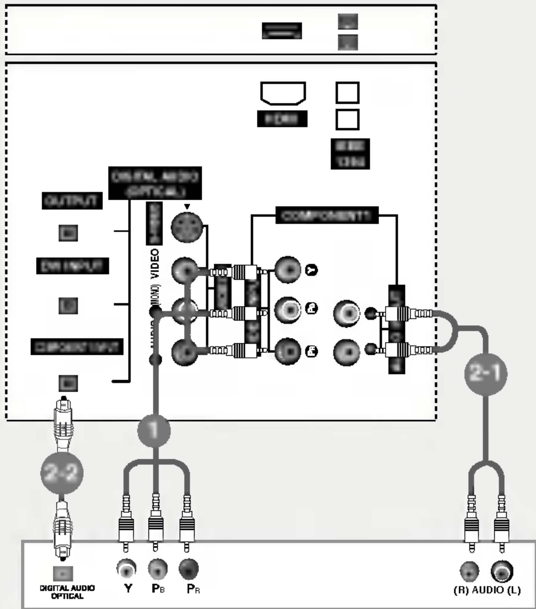
Boîtier décodeur numérique
