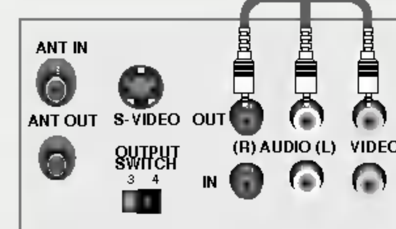
VCR (magnétoscope)
