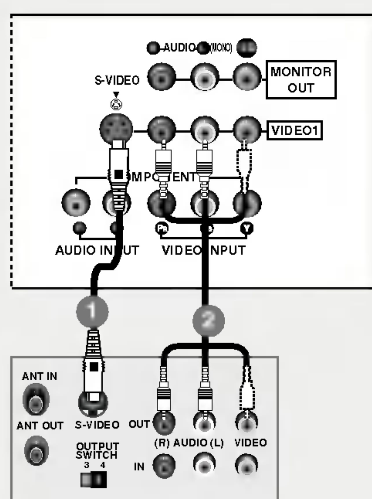
VCR (magnétoscope)
