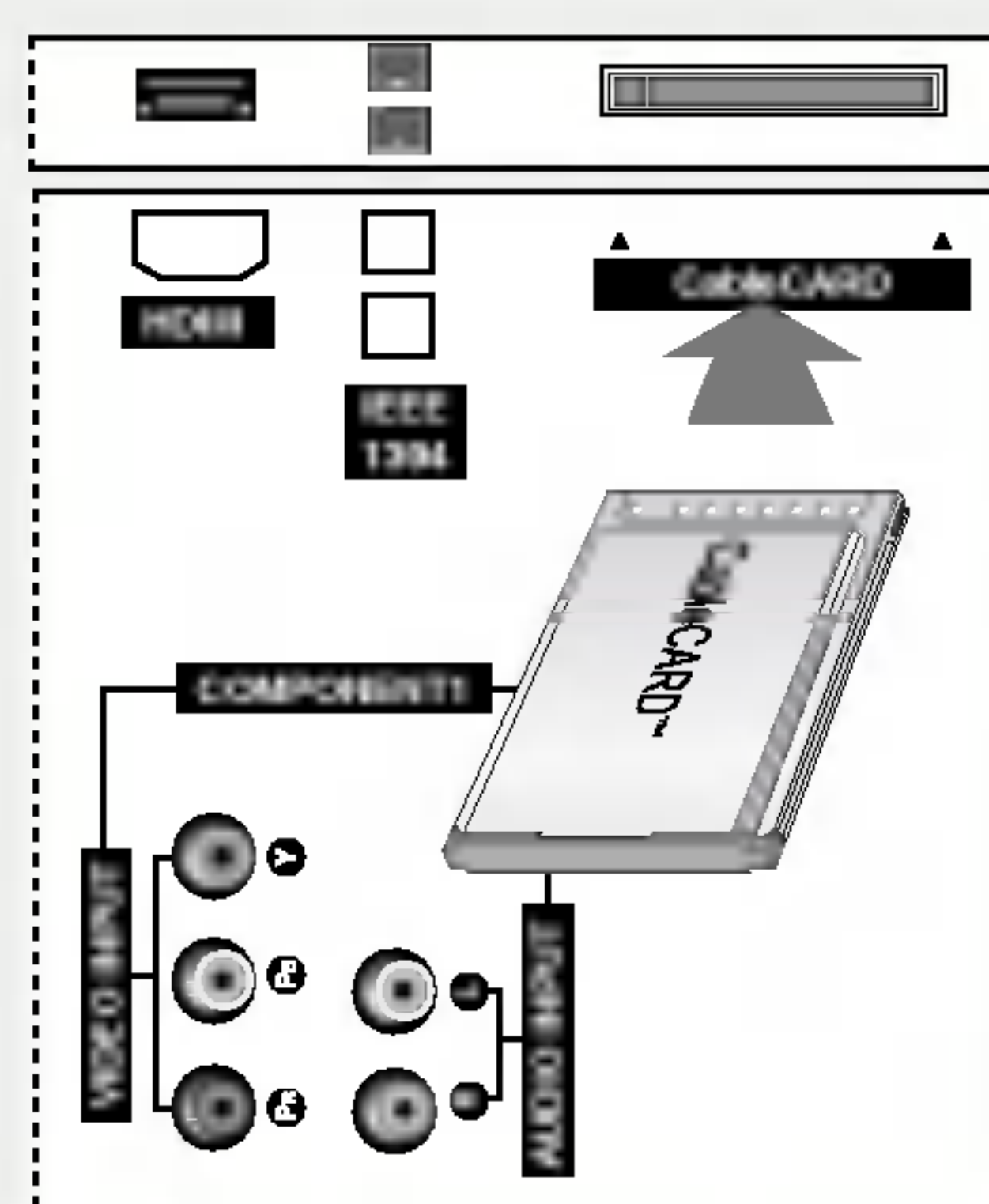
Arrière du téléviseur de 26 pouces
