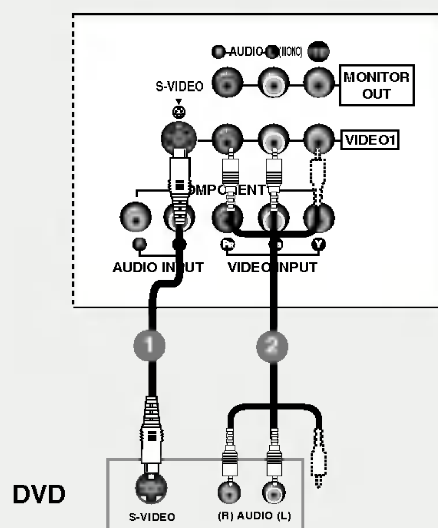
Arrière du téléviseur de 32, 37 et 42 pouces
