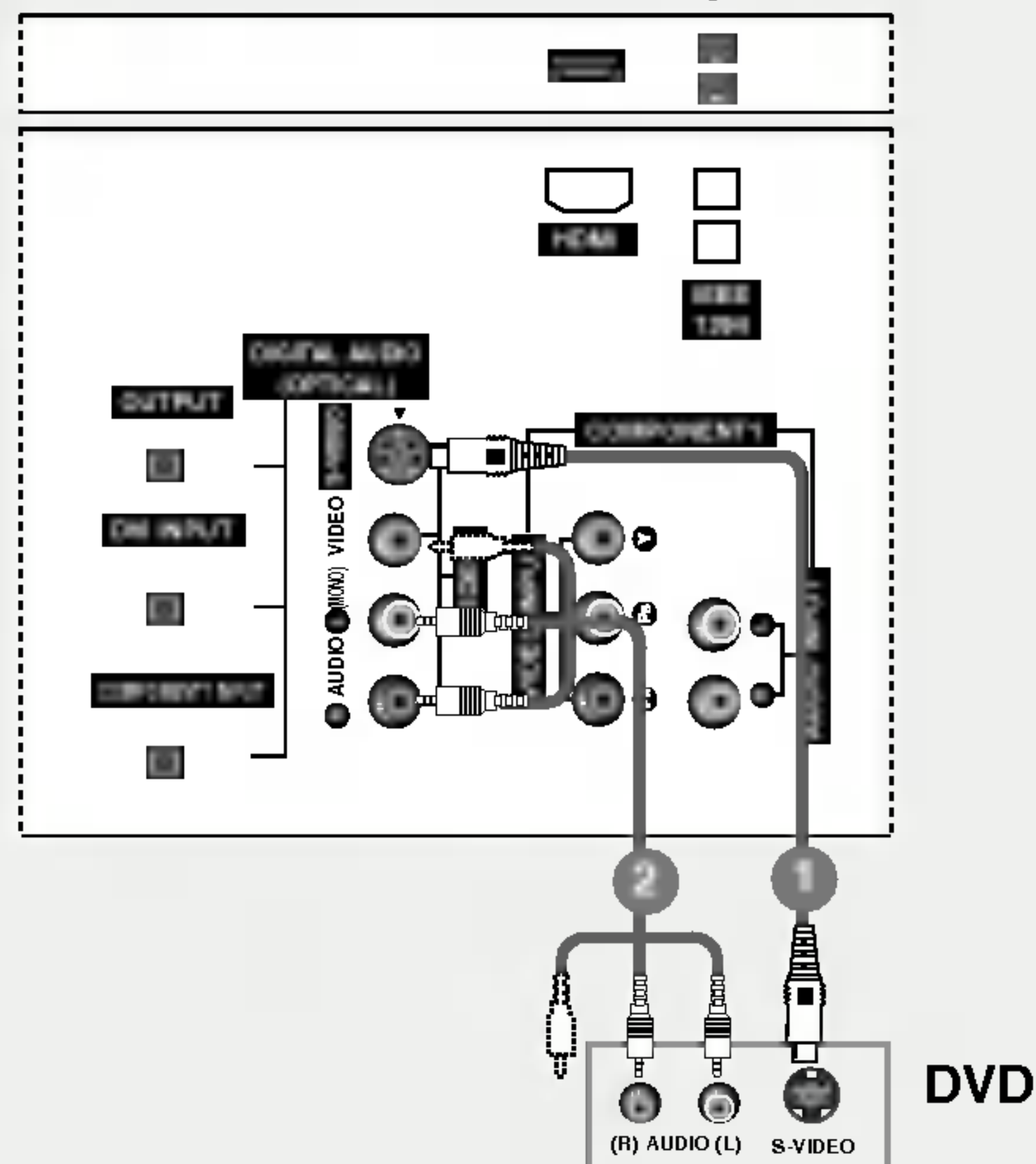
Arrière du téléviseur de 26 pouces
