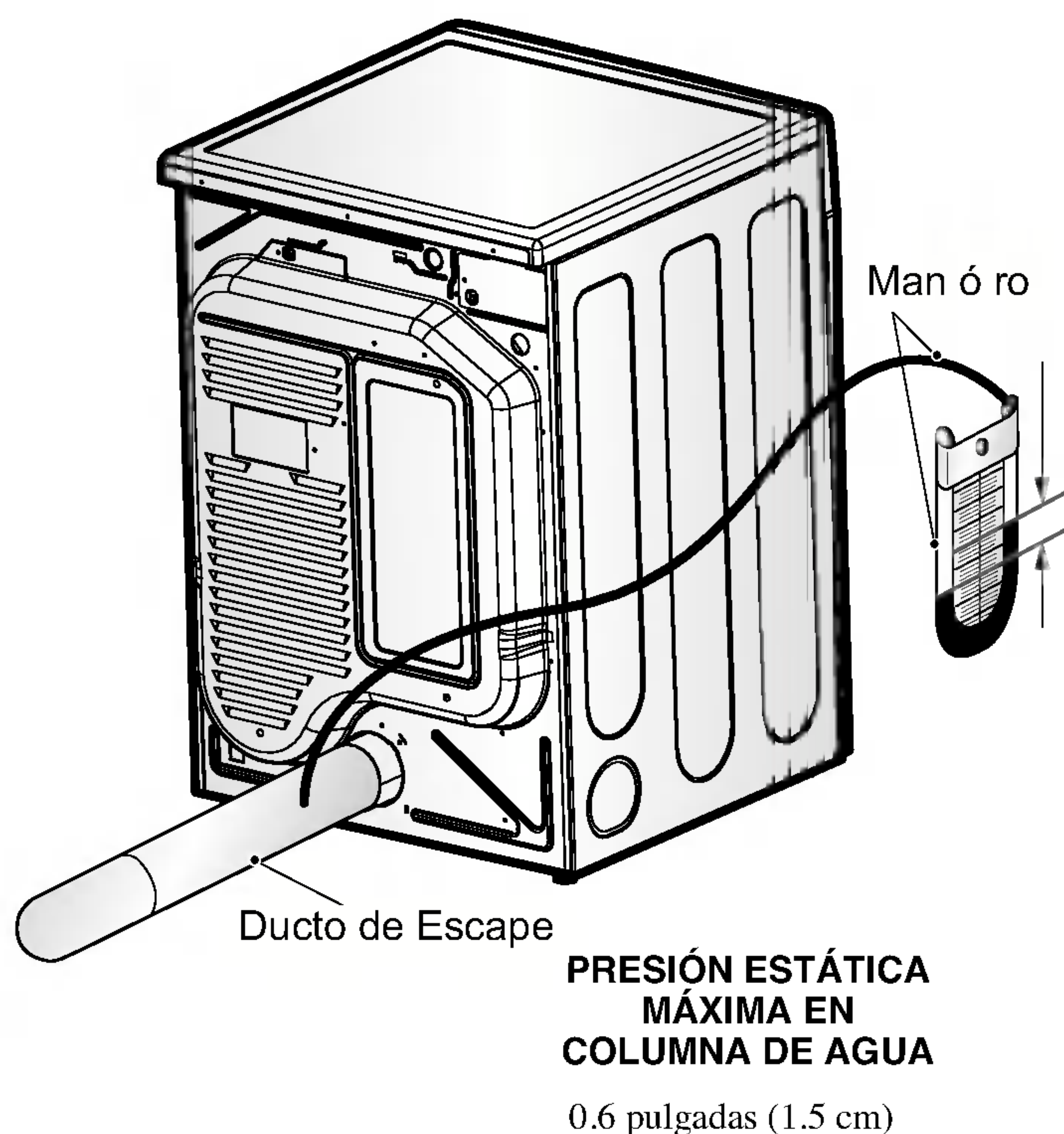
Medición de la Presión Estática.
