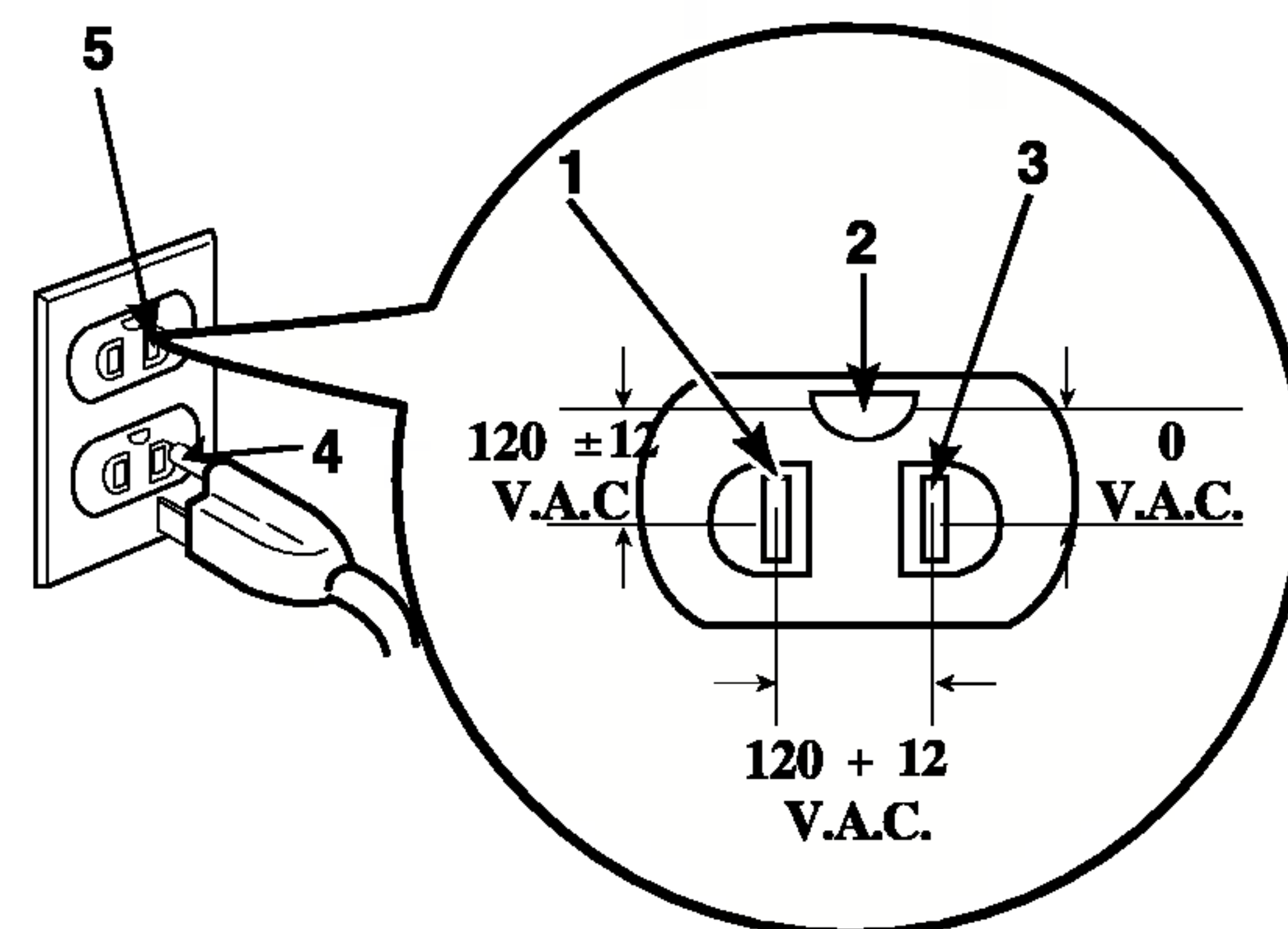
CIRCUITO ESTÁNDAR DE 127 VOLT, 60 HERTZ, 3-ALAMBRES EFECTIVAMENTE CONECTADO A TIERRA.
