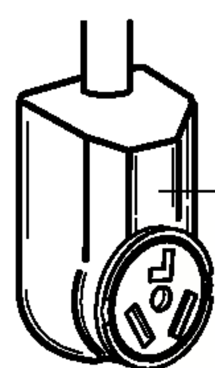
Enchufe de 3-alambres Terminales de espada con puntas levantadas Clavija neutral
