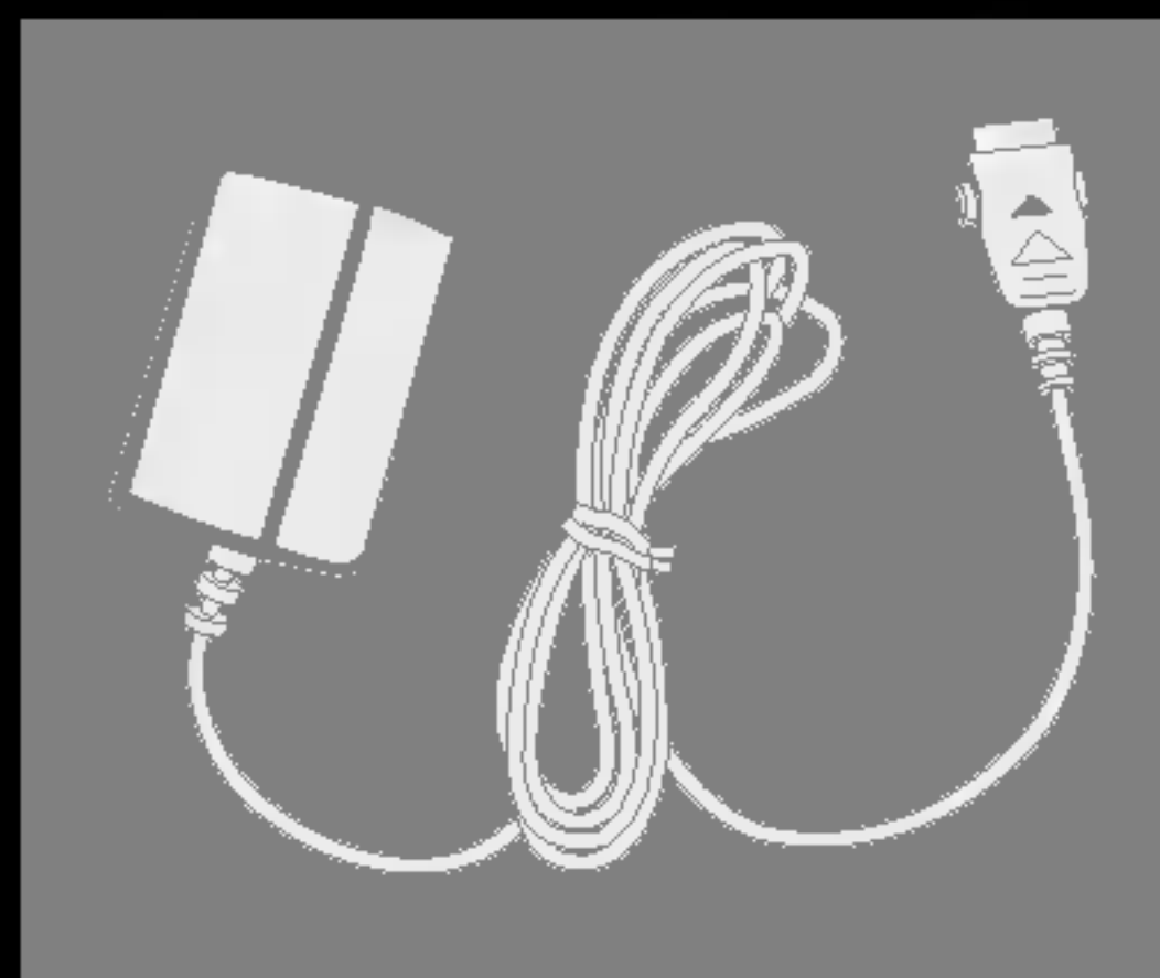
Adaptador para viajes Especificaciones: Entrada: 100-240 V~50/60 Hz 150-100 mA Salida: 5,2 Vcc 800 mA
