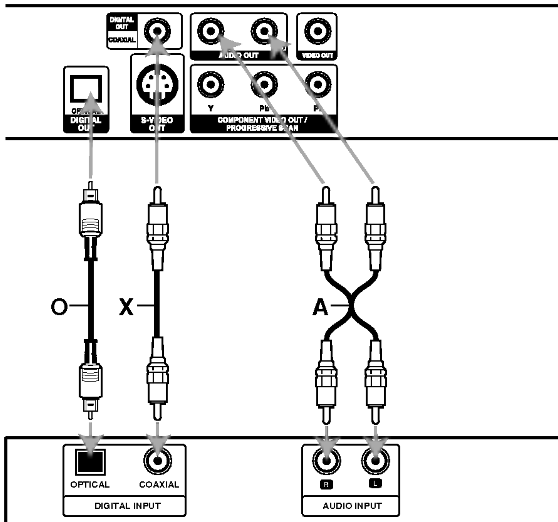
Усилвател (приемник)
