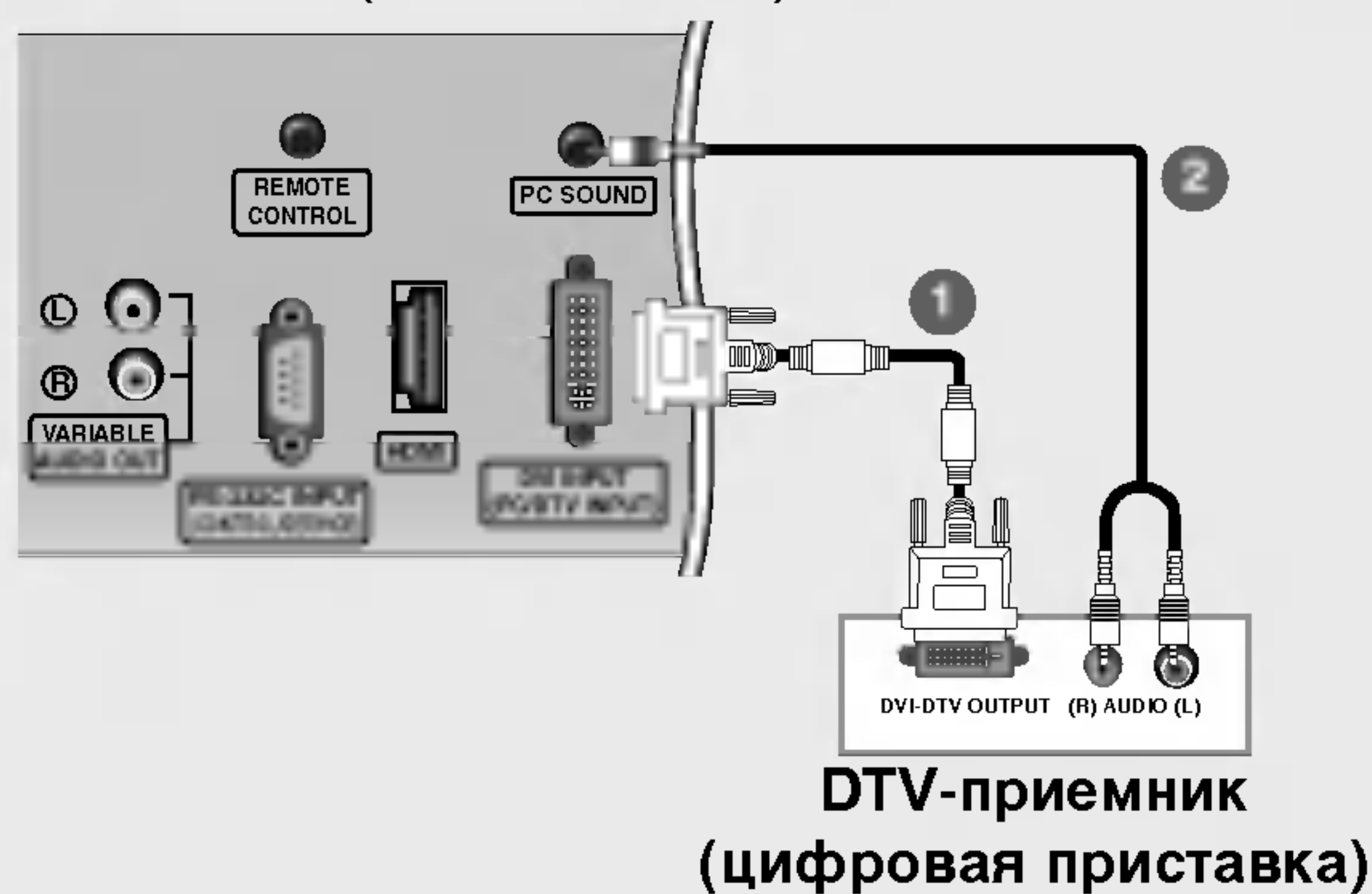
Задняя панель ТВ (32 дюйма или 81 см)
