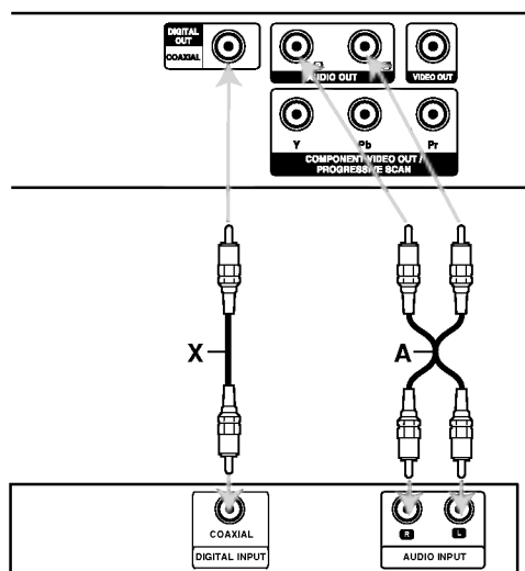
Zosilňovač (Prijímač)
