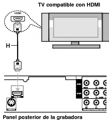
Panel posterior de la grabadora
