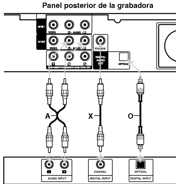
Amplificador (Receptor)
