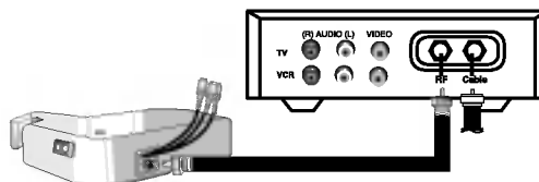
Panneau de connexion de la boîte de raccordement.
