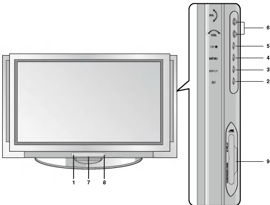
< Panel czołowy >
